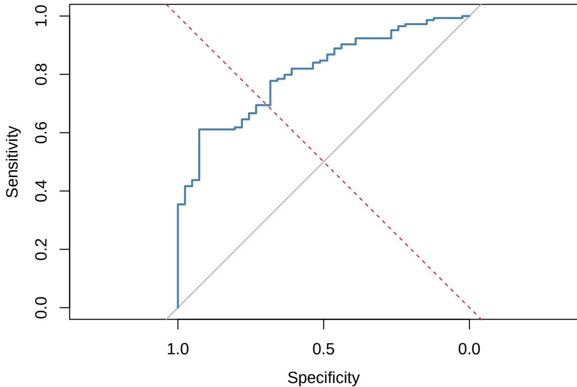
Curva ROC – Modelo Logístico
