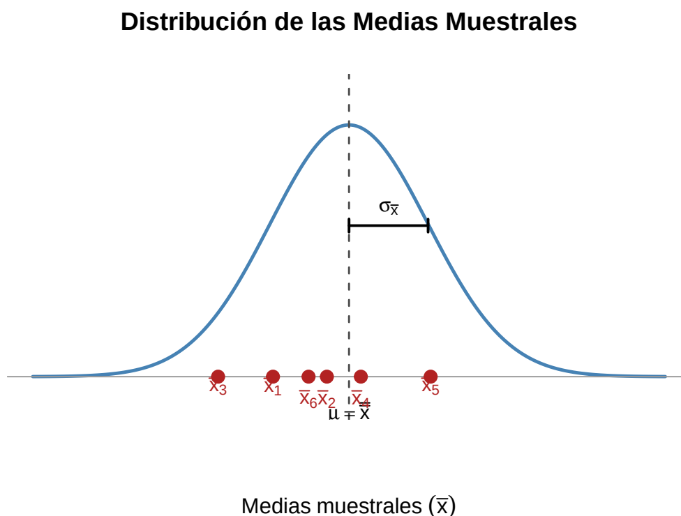
Figura 1.2: Teorema del Límite Central
