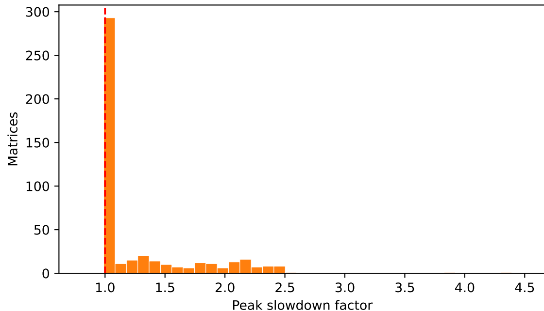
Intel MKL SpMV (n=460) 174 (38%) anomalous
