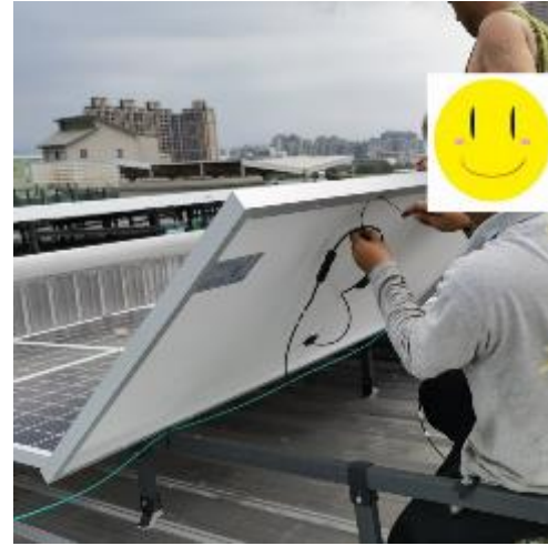
模組鋪板及串線
