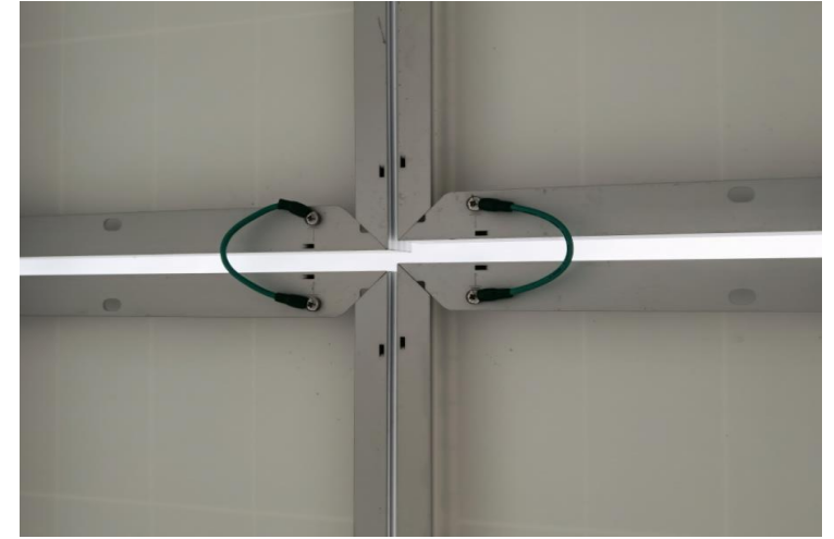
模組接地線串接
