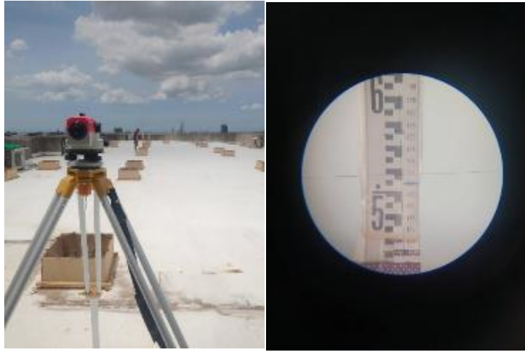
水泥墩座放樣
