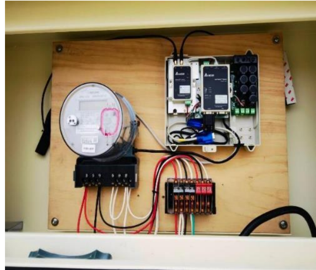
台電電表安裝接線
