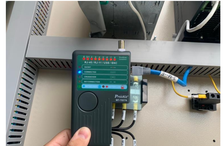
監控線路測試
