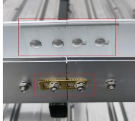
鋁線槽安裝
