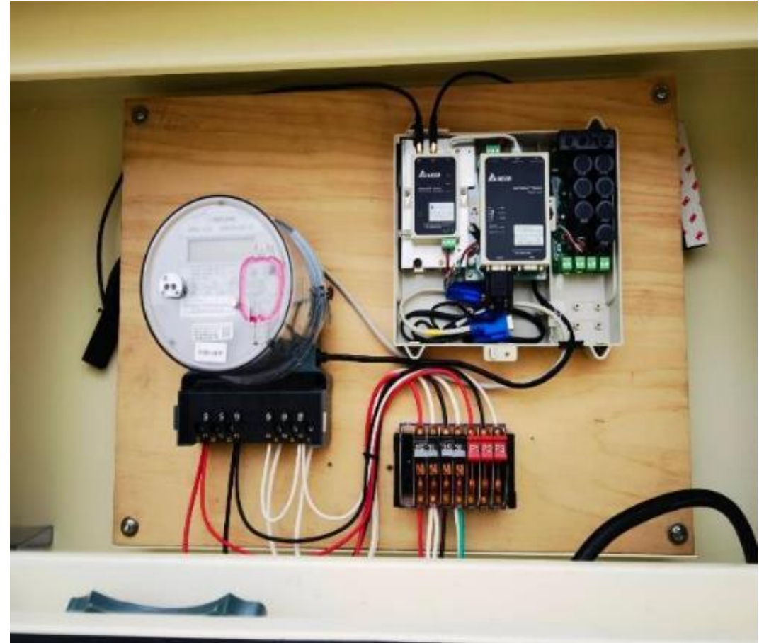
台電電表安裝接線
