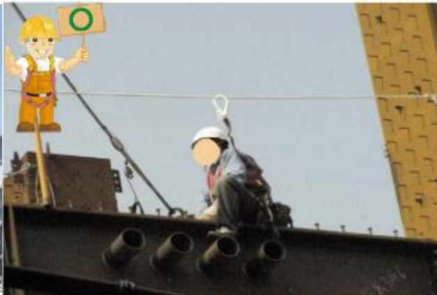
圖 42 勞工已確實配掛荷負式安全帶並鉤掛於水平母索
