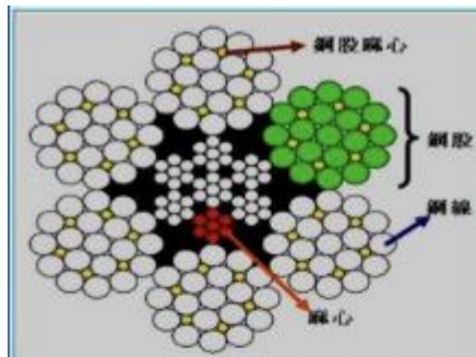
圖3 CNS941填充型6股25線鋼纜圖
