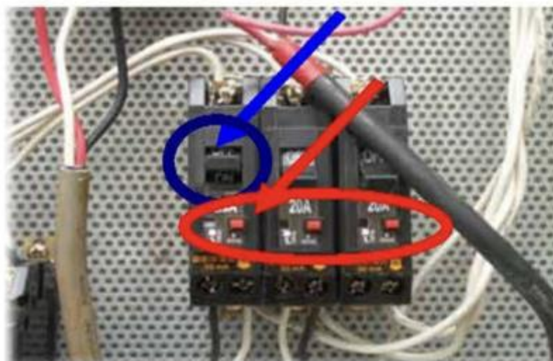
漏電斷路器押下測試鈕（ 紅色箭頭所指之處）後跳 脫情形。
