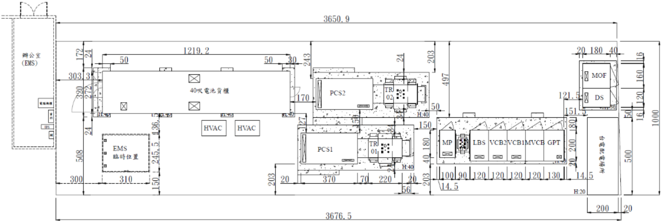
1 GL001 儲能設備平面配置圖
