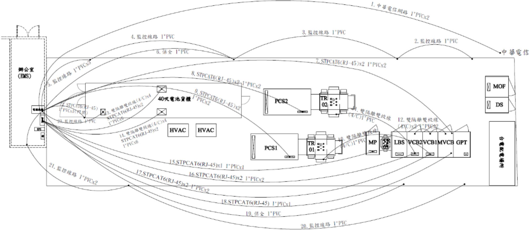
1 GL006 通訊及控制管線配置圖
