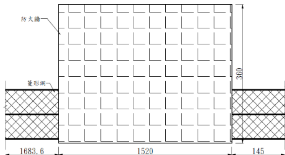
3 圍籬與防火牆示意圖
