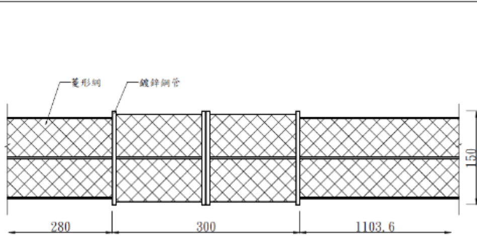
2 圍籬對開門立面圖
