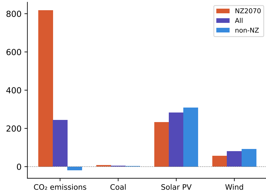
ME
