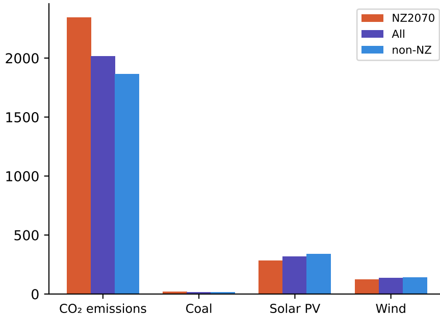
MAE
