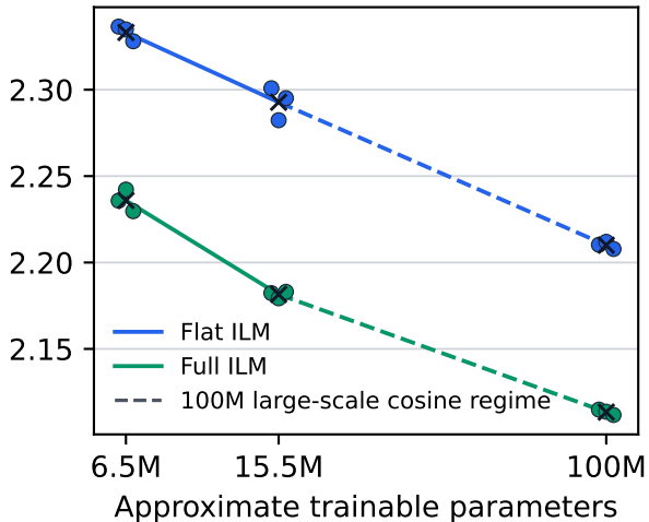
enwik8
