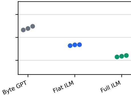
enwik8
