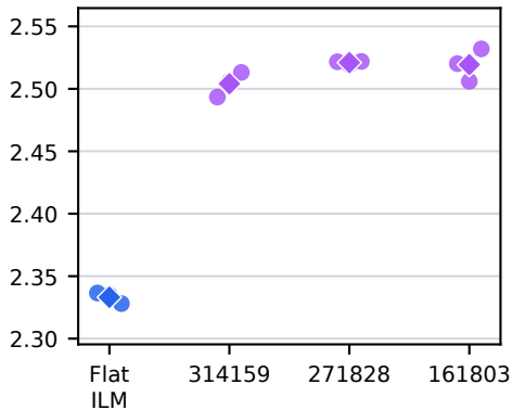
enwik8
