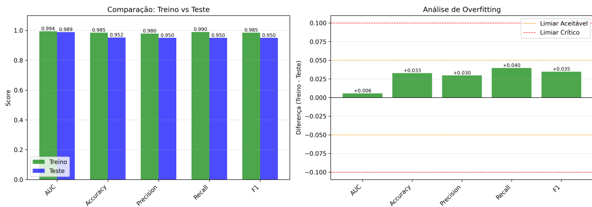
Figura 5 – Análise de sobreajuste: comparação entre métricas de treino e teste do modelo LightGBM.
