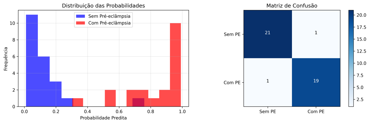
Figura 4 – Distribuição de probabilidades previstas e matriz de confusão do modelo LightGBM.
