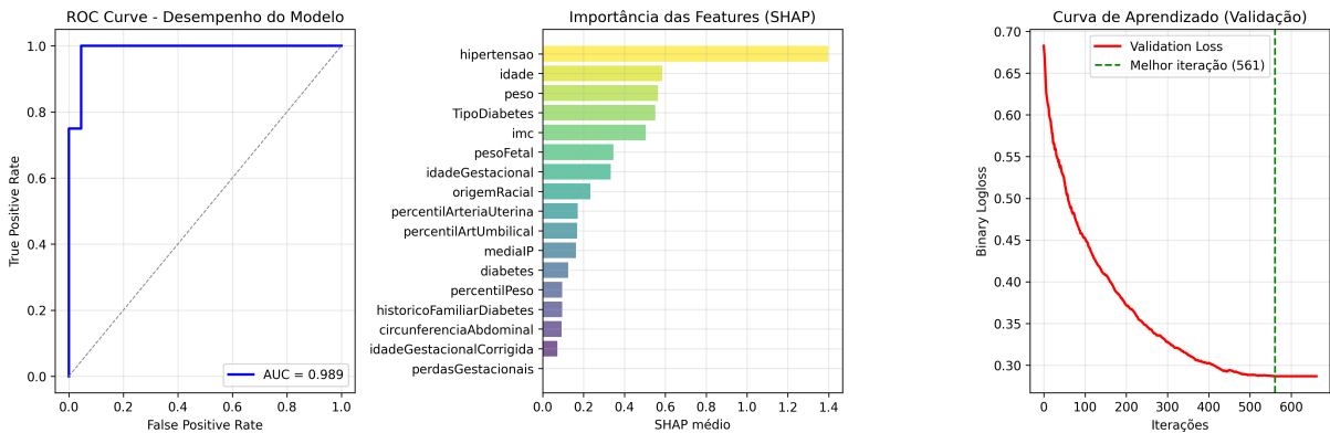
Figura 3 – Métricas de avaliação do modelo LightGBM: curva ROC, importância das variáveis e curva de aprendizado.
