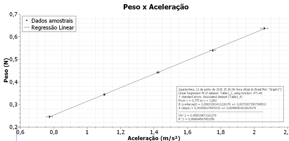
Figura 1: Regressão linear do peso suspenso p em função da aceleração a do sistema (Parte 1). O coeficiente angular corresponde à massa total (M + m) .
