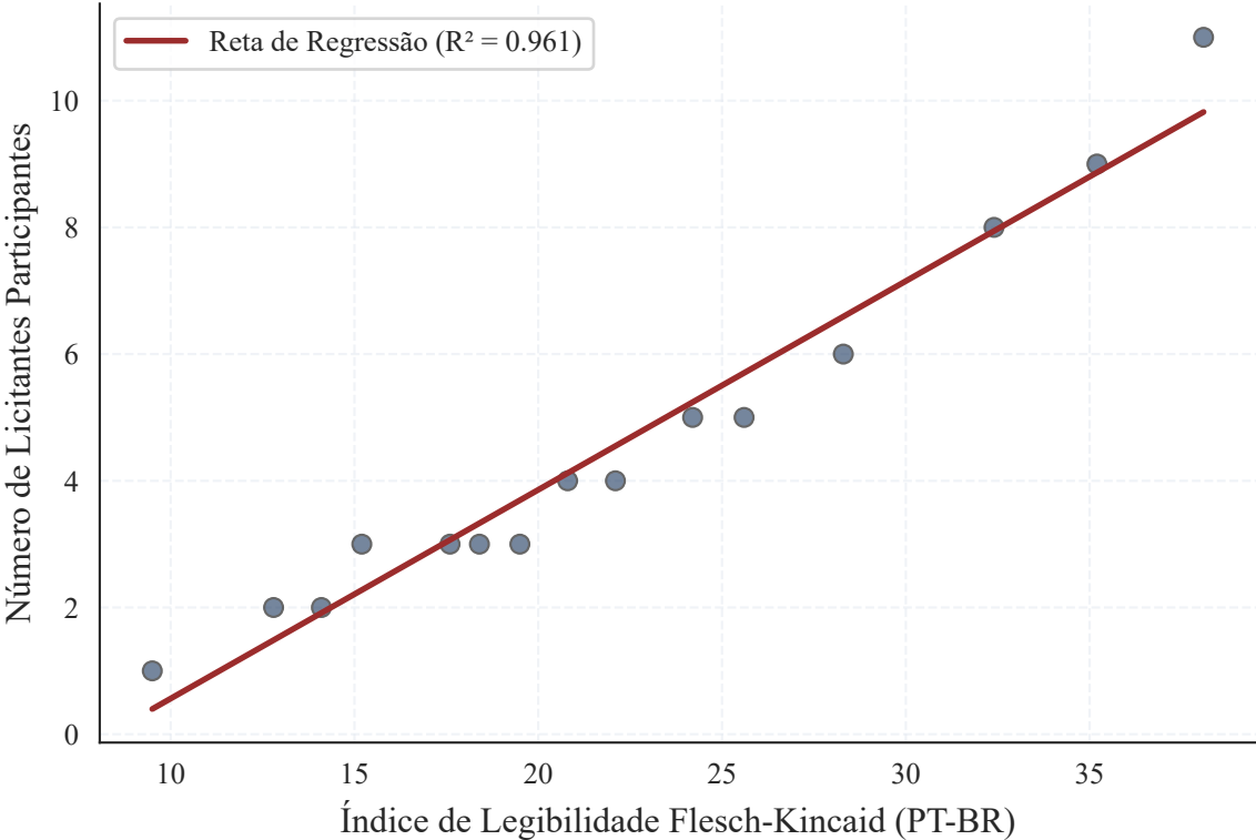
Figura 1 - Correlação entre Facilidade de Leitura (Flesch-Kincaid) e Número de Licitantes
