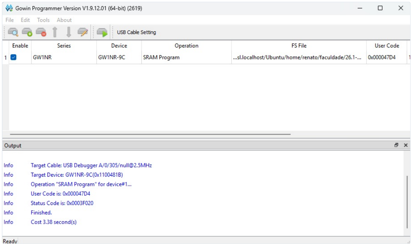
Figura 7 - Programacao SRAM concluida no Gowin Programmer. A janela mostra Finished e tempo de programacao de 3,38 s.
