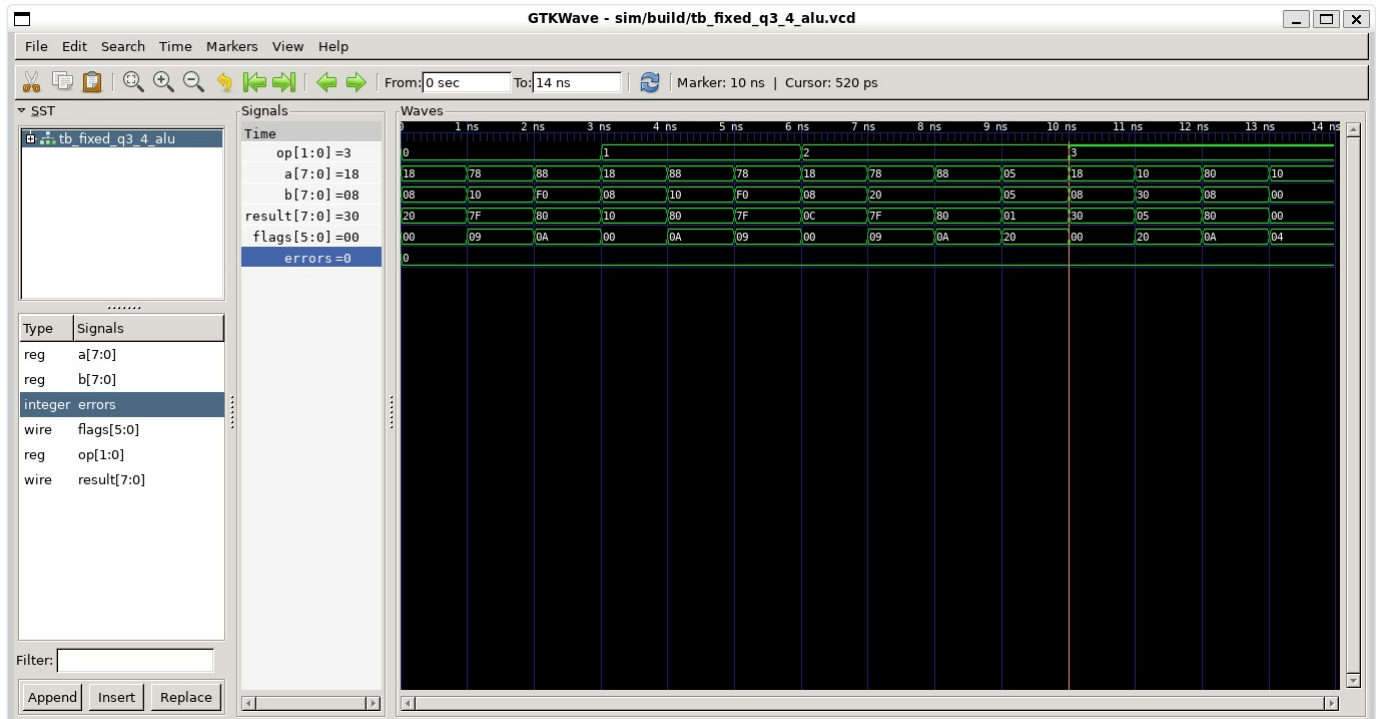
Figura 2 - Ponto fixo Q3.4 com saturacao positiva/negativa e truncamento. As flags 09, 0A e 20 evidenciam saturacao e inexatidao.
