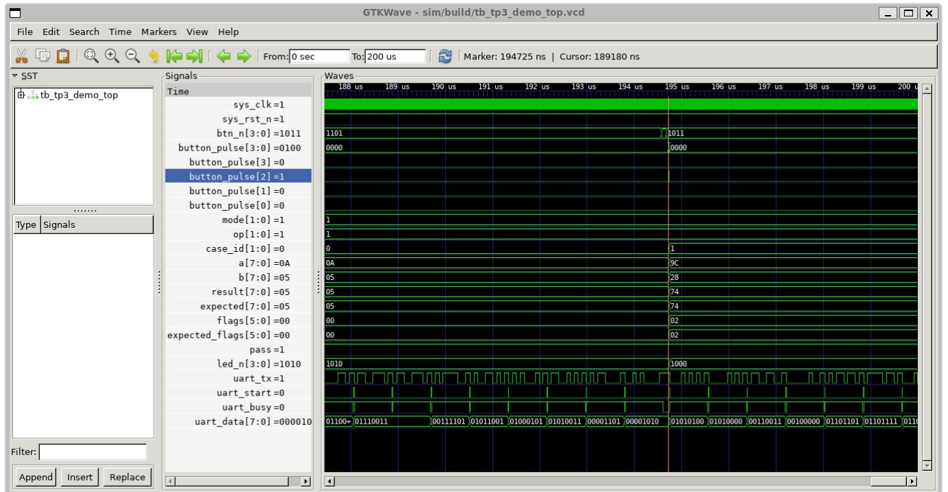
Figura 4 - Top de demonstracao com pulso em button_pulse[2] , mudanca de caso para case_id=1 , atualizacao de flags, LEDs e atividade UART.
