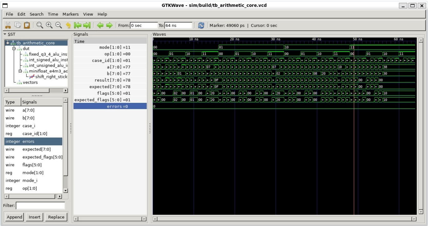
Figura 1 - Core integrado percorrendo modos, operacoes e casos. O print mostra resultado igual ao esperado, flags iguais as esperadas e contador de erros em zero.
