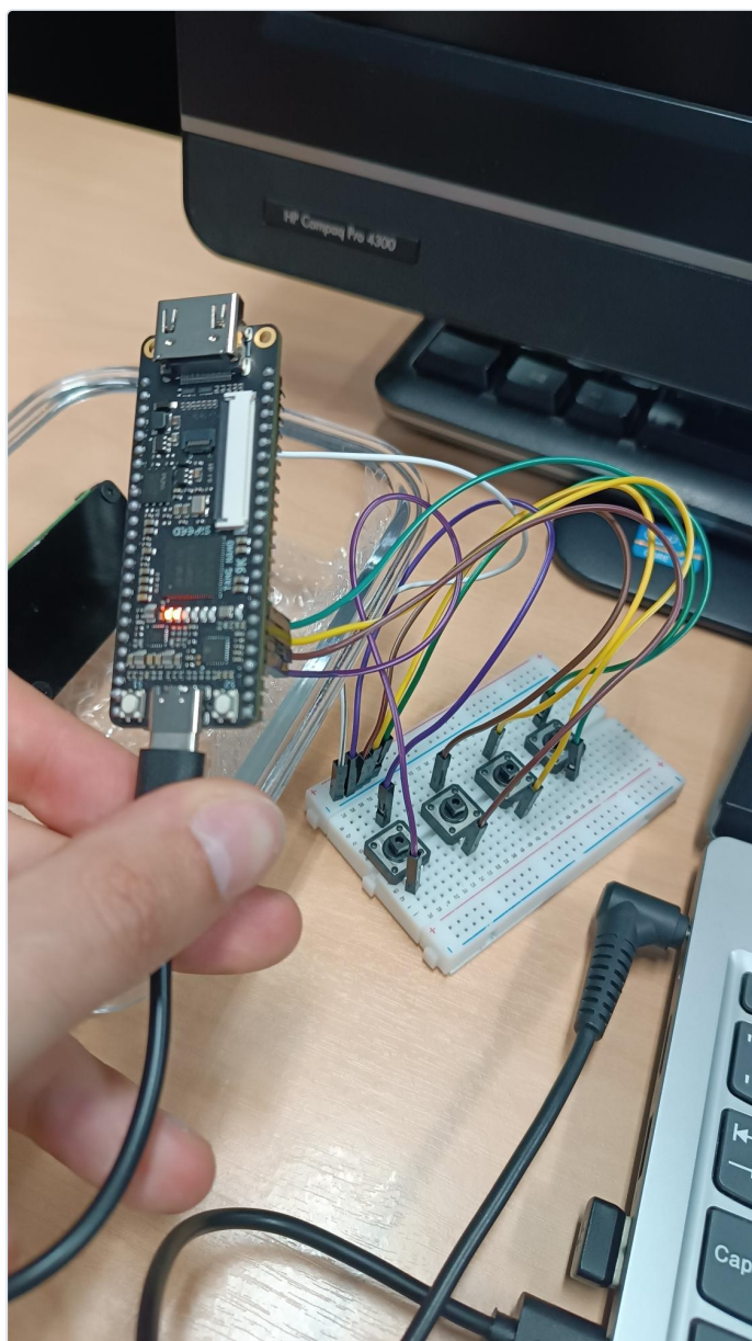
Figura 8 - Montagem fisica com a Tang Nano 9K, quatro botoes externos no protoboard e GND comum.
