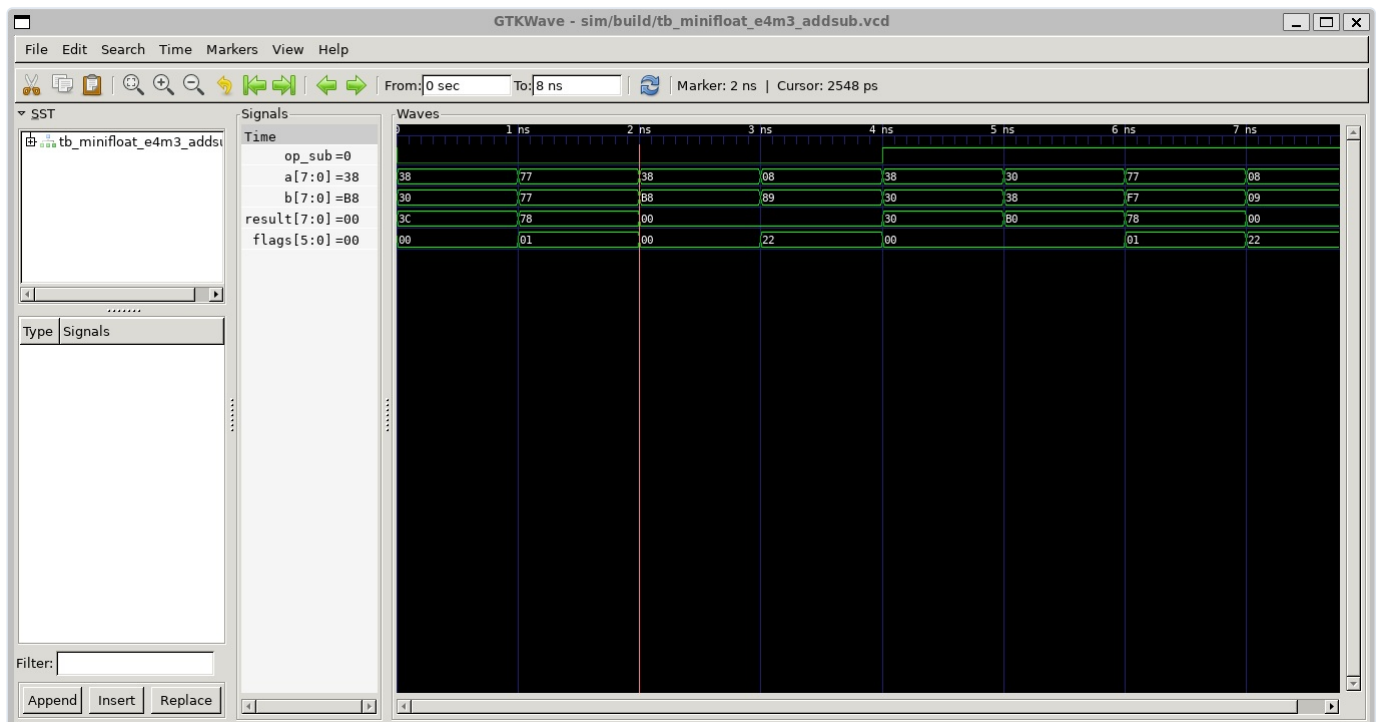
Figura 3 - Ponto flutuante simplificado E4M3. A simulacao mostra overflow para infinito com result=78 flags=01 e underflow para zero com result=00 flags=22.
