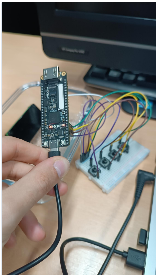
Figura 10 - Estado inicial apos reset: caso UINT8 ADD case=0, sem flags e PASS ativo.
