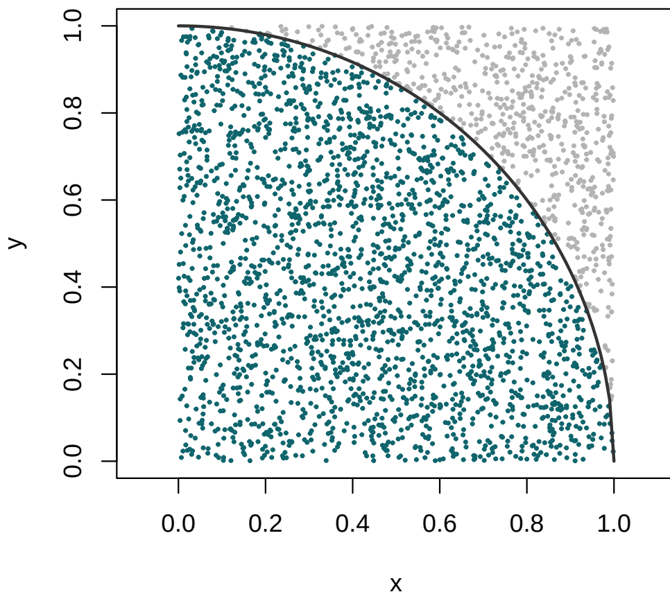
Figura 25.2: Estimativa de \pi pelo método acerta-ou-falha: pontos aleatórios no quadrado unitário. Os que caem dentro do quarto de círculo (a azul) representam uma fração próxima de \pi/4 .
