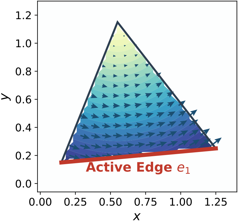
(d) FEM Whitney 1-Form w_1(x)
