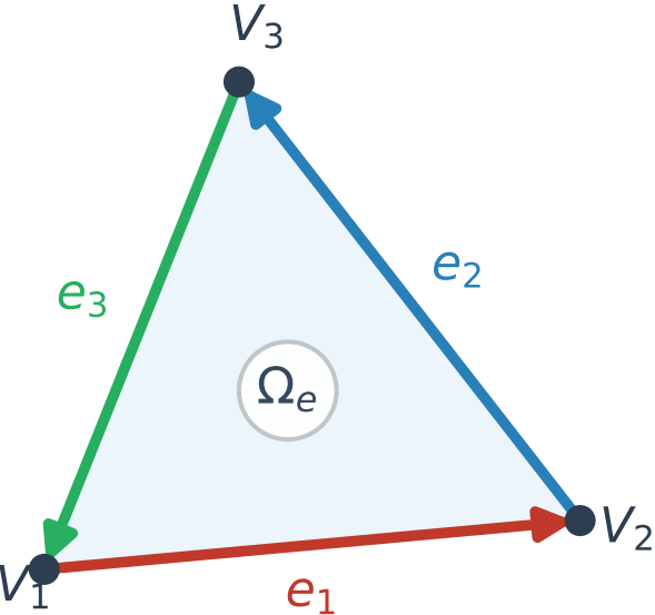
(a) FEM Whitney Edge Element
