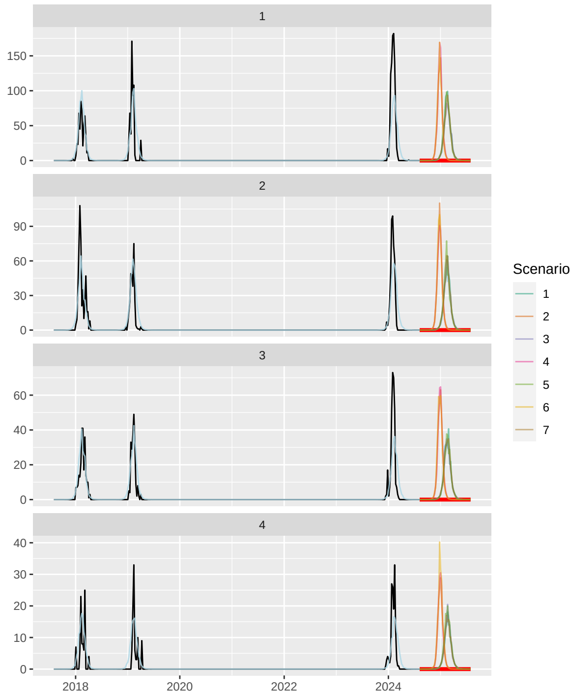
Slovenia (SI), ILI incidence
