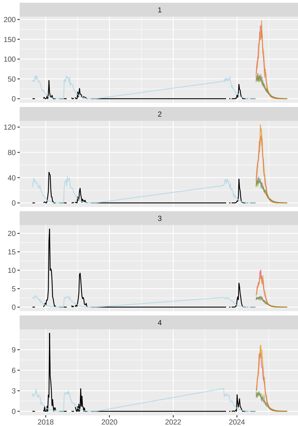
Romania (RO), ILI rate
