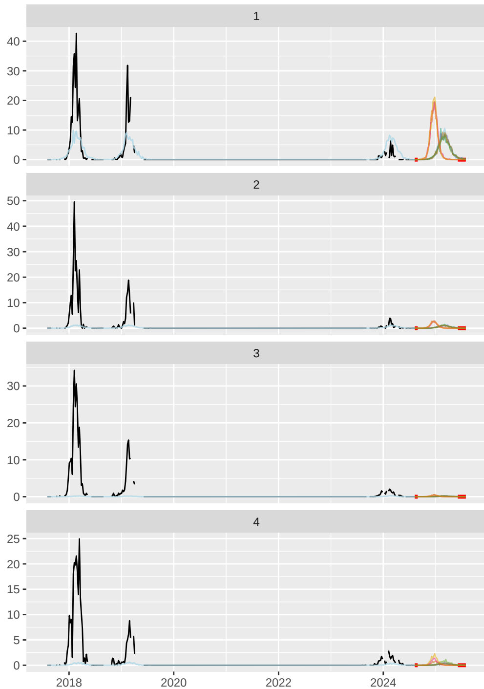
Iceland (IS), ILI rate
