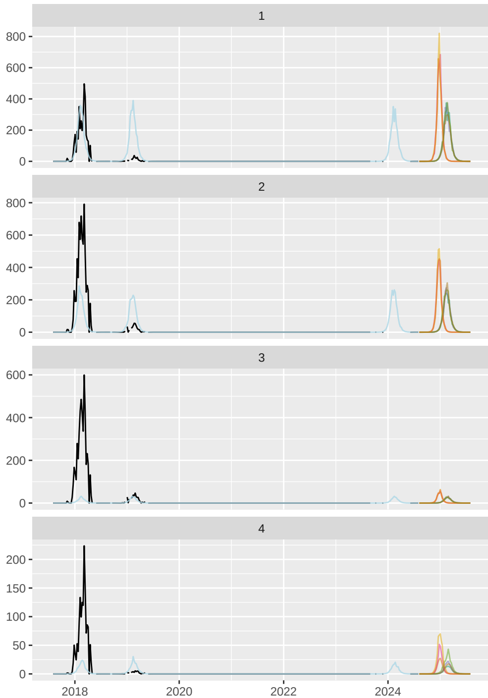
Finland (FI), ILI rate
