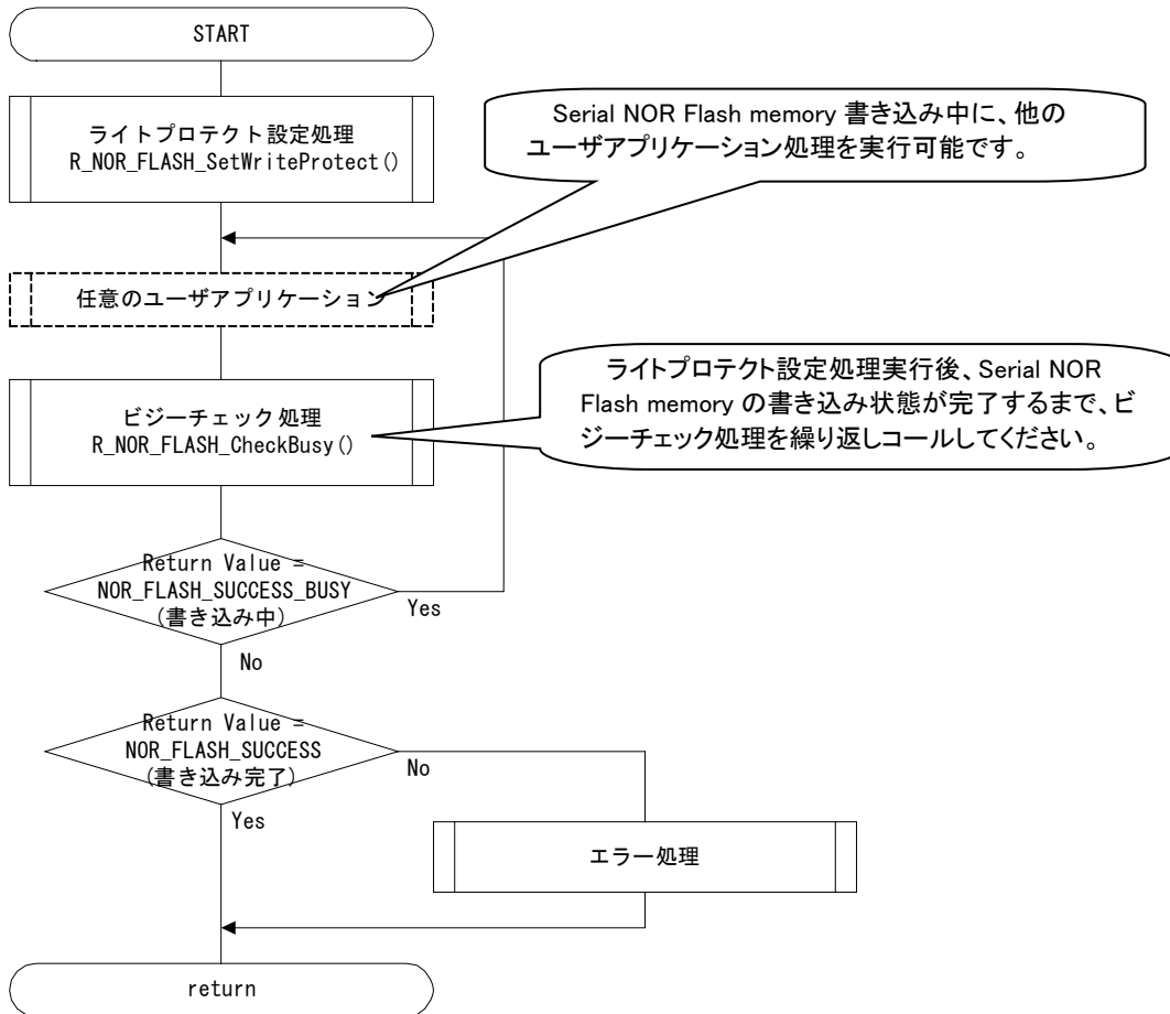
図 3-1 R_NOR_FLASH_SetWriteProtect()の処理例
