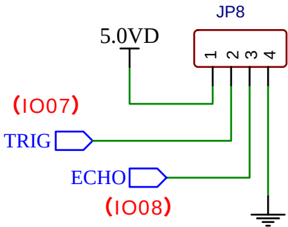
超声波插座
