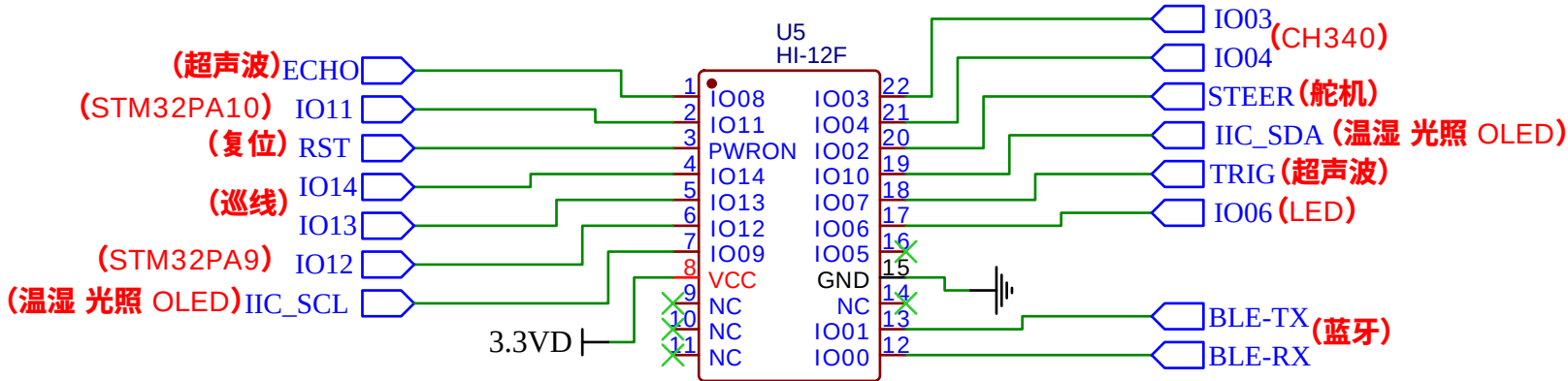
Hi-3861 模块
