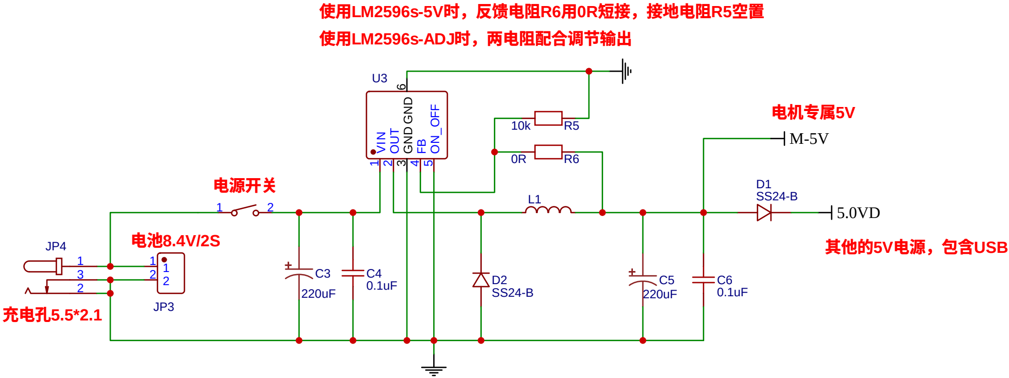
电源 DC-DC 5V
