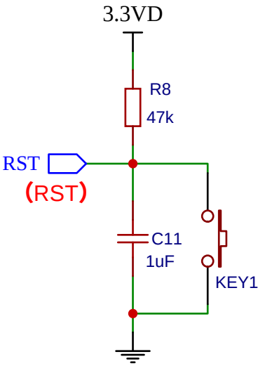
复位电路
