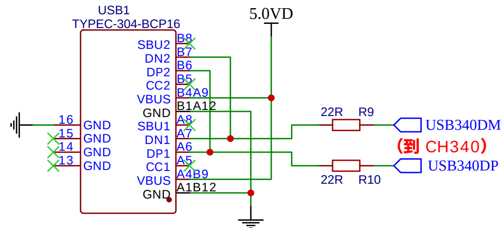
TYPE-C接口(外壳单点接地)
