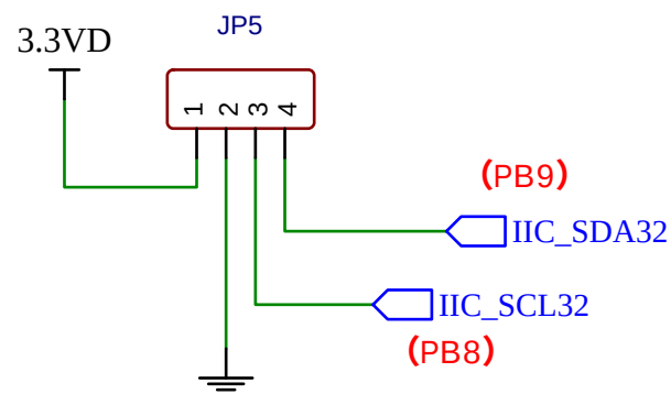
陀螺仪，加速度传感器
