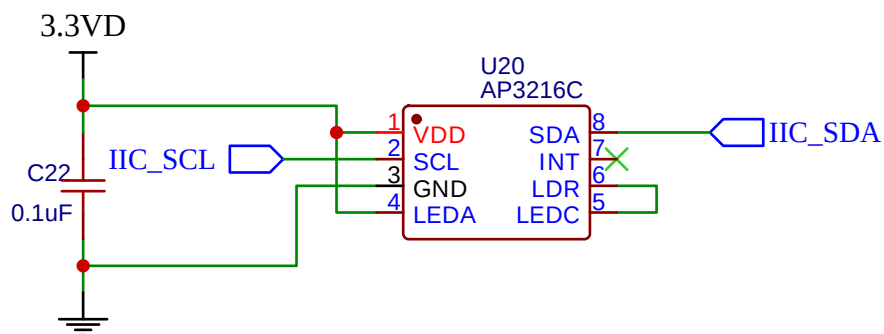
环境光传感，接近传感器（0x1E）
