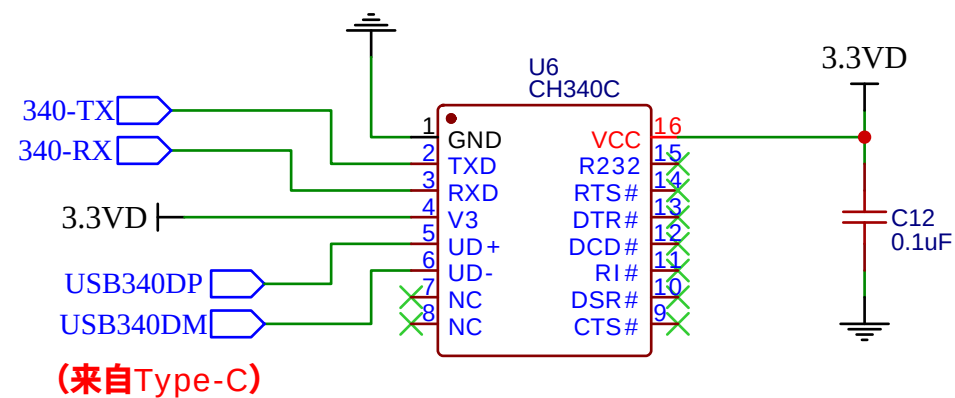
USB转串口
