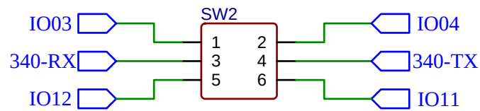
USB 串口切换
