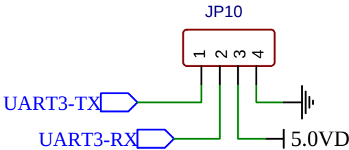
串口输出
