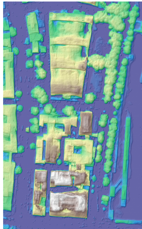
(d) Fractional feathering: roof detail
