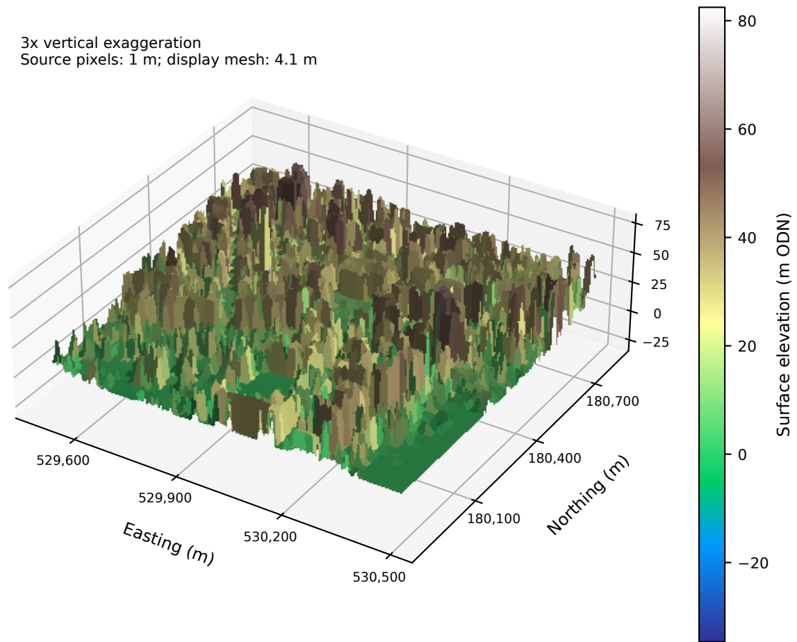
(b) Oblique DSM
