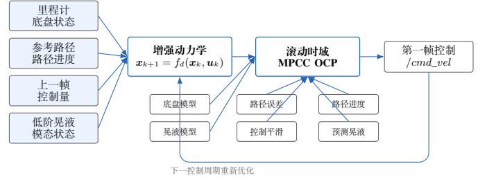
Fig. 2. SPMPC 增强状态与 OCP 结构。规划器将底盘状态、路径进度和低阶晃液状态放入同一预测模型, 在滚动时域内联合考虑路径跟踪、路径推进、控制平滑和预测晃液响应, 并只执行第一帧底盘命令。
