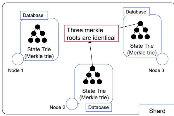
图 11.1: 同一个分片的共识节点通过验证状态树的 merkle root，来判断区块是否正确。
