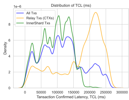
图 4.8: 实验图：不同类型的交易时延的统计。
