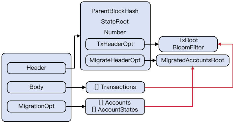
图 7.4: 区块的新数据结构。
