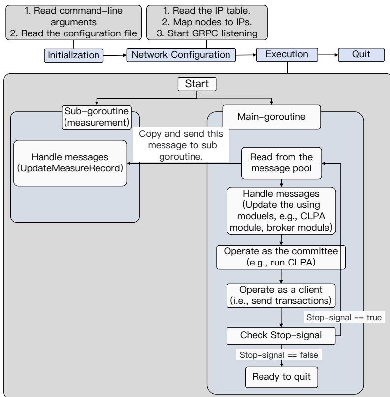
图 7.2: Supervisor 节点在 BE-X 中的工作流程。
