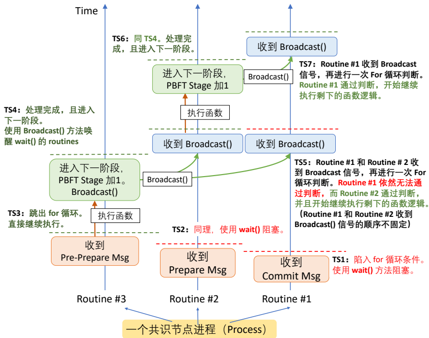
图 9.1: 使用 Go Routine 解决 PBFT 消息乱序的方案。图中的 TS 是 time stamp 的缩写, 表示事件发生的时间。
