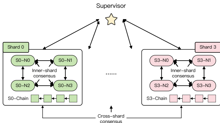
图 7.1: BE-X 的系统架构, 图中的部署规模为 4 \times 4 + 1 (共 4 个分片, 每个分片 4 个共识节点, 还有一个 supervisor 节点)。
