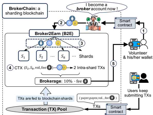
图 6.1: Broker2Earn 协议在 BrokerChain 分片区块链中的工作原理。
