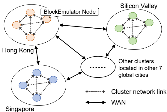
图 11.4: 多机部署 BlockEmulator 的例子。其中 Hong Kong 虚拟机的 IP 地址为 10.1.1.10, Singapore 虚拟机的 IP 地址为 10.2.2.20, Silicon Valley 虚拟机的 IP 地址为 10.3.3.30。
