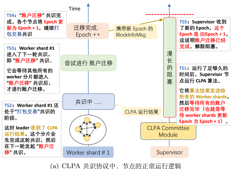
(a) CLPA 共识协议中，节点的正常运行逻辑
