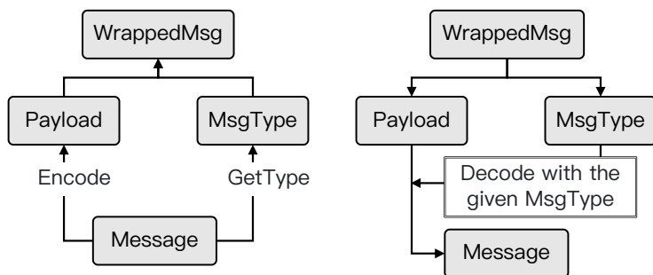
图 7.6: WrapMsg 的编码与解码逻辑。
