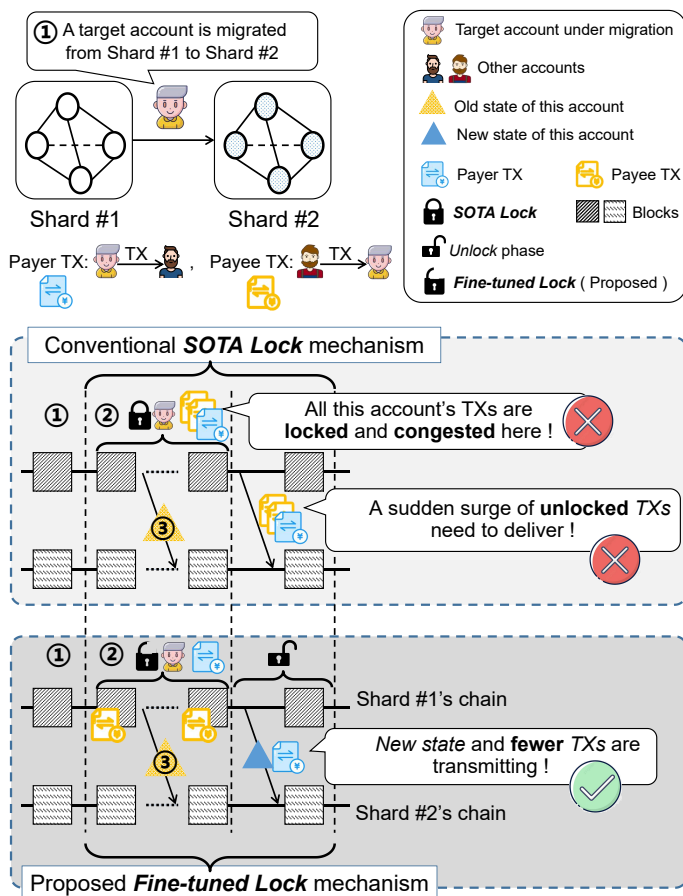
图 5.2: SOTA Lock 与 Fine-tuned Lock 机制之间的对比。①：触发账户迁移，一个目标账户从 shard #1 迁移至 shard #2。②：锁操作开始。③：将被迁移账户的旧状态数据发送到 shard #2。
