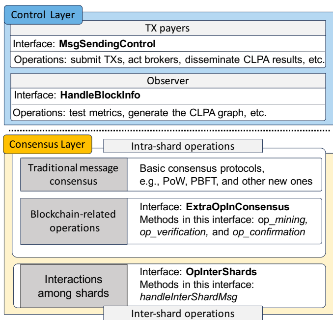
图 11.3: BlockEmulator 的接口设计。
