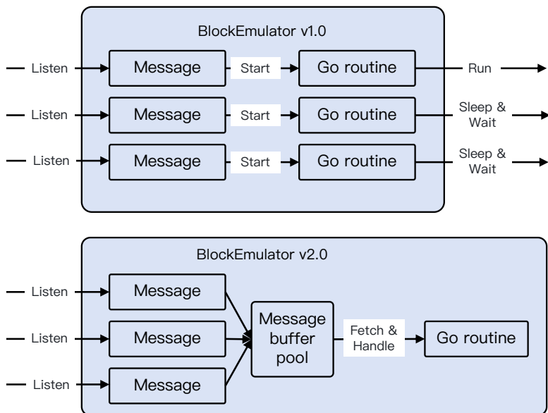
图 7.7: BE v1.0 与 BE v2.0 对节点执行中的消息处理逻辑对比。
