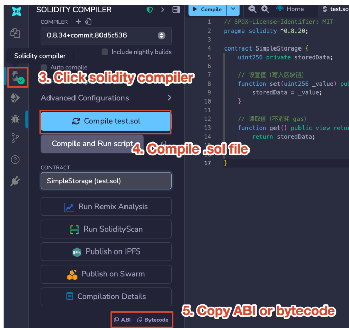
图 8.4: 使用 Remix 编译智能合约。
