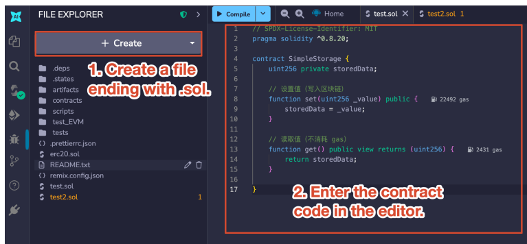
图 8.3: 使用 Remix 编写智能合约。
