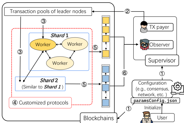
图 2.2: BlockEmulator 的主要角色，与内部工作流程。
