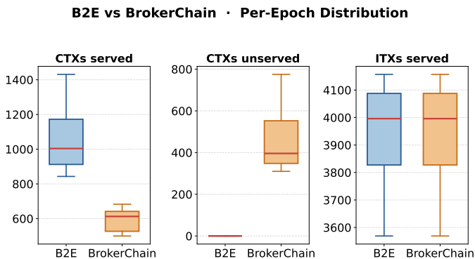
图 6.5: B2E 以及 BrokerChain 的性能表现。其中，CTXs: cross-shard TXs; ITXs: intra-shard TXs。
