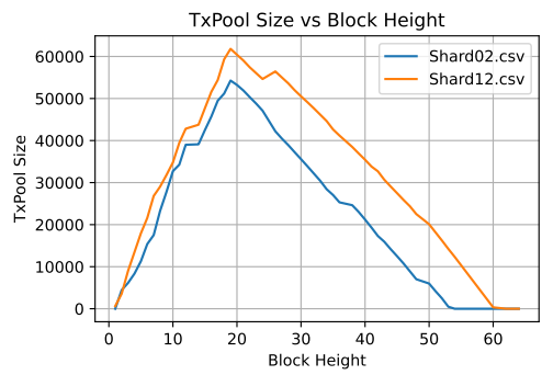
图 4.9: 实验图：交易池的动态变化。
