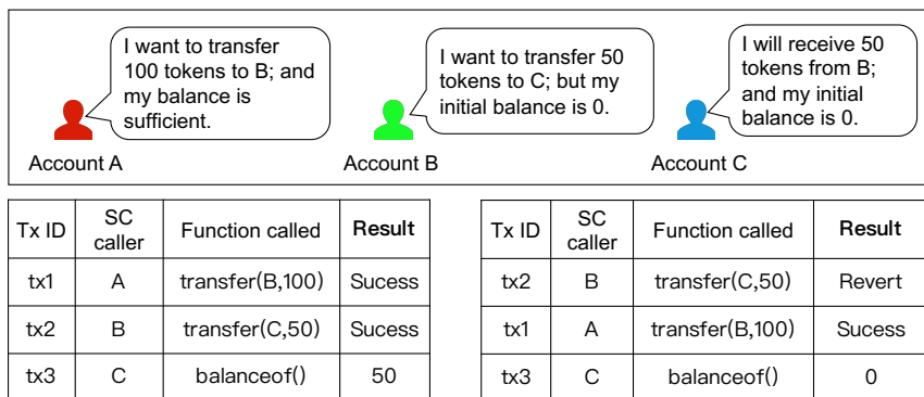
图 8.1: “交易顺序敏感性”的案例示例。图中 SC 代表 Smart Contract。
