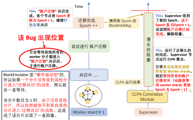
(b) CLPA 协议触发这个 bug 的原因。
