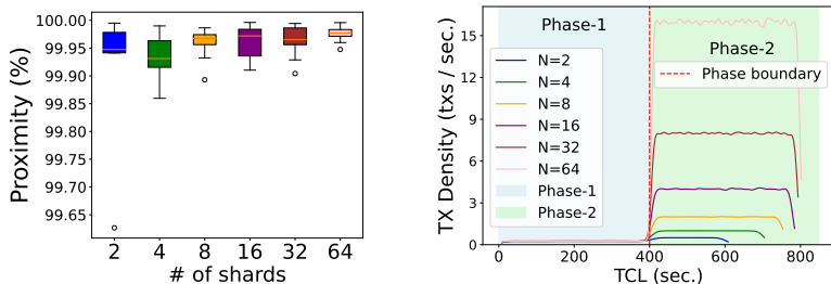
(a) BlockEmulator TPS 的实验结果与理论推导的接近程度 (%)。
