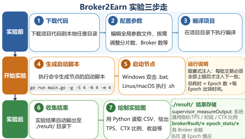
图 6.2: Broker2Earn 实验完整操作流程概览。
