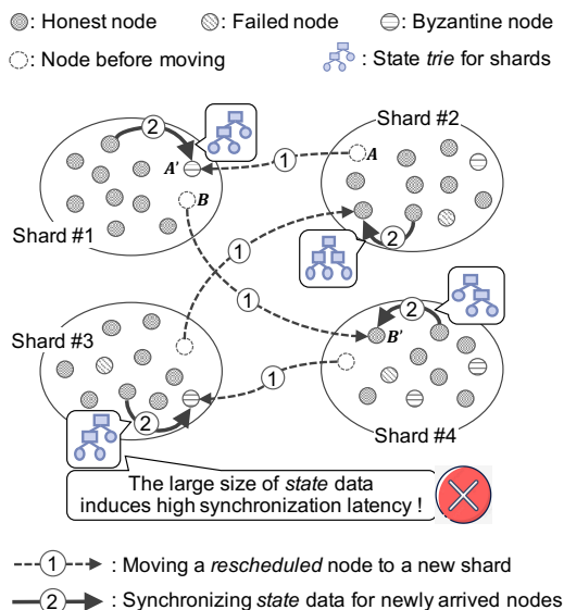
图 5.3: 系统进行分片重组操作时, 每个分片内一部分共识节点会被迁移到其他分片。问题是: 在对某个节点进行跨分片迁移时, 如何支持对新加入节点本地维护的状态数据进行更新。当需要被同步的数据量太大时, 数据同步操作会导致分片重组耗时太久。
