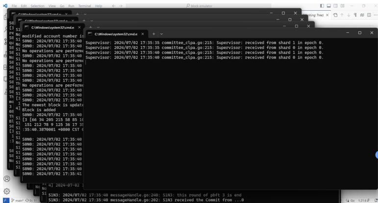
图 4.5: 运行 blockEmulator。
