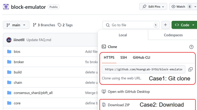
图 4.1: 下载 blockEmulator。
