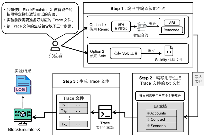
图 8.2: 使用 BlockEmulator-X 进行智能合约测试的流程概览图。
