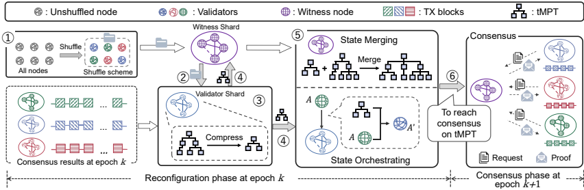
图 5.4: tMPT 协议的运行流程。
