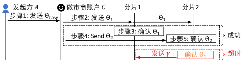
图 2.5: BrokerChain 协议中跨分片交易处理流程。
