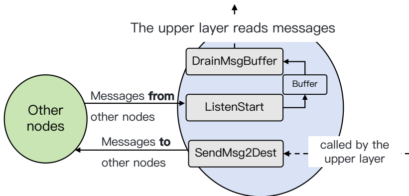
图 7.5: 消息缓冲区的设计。
