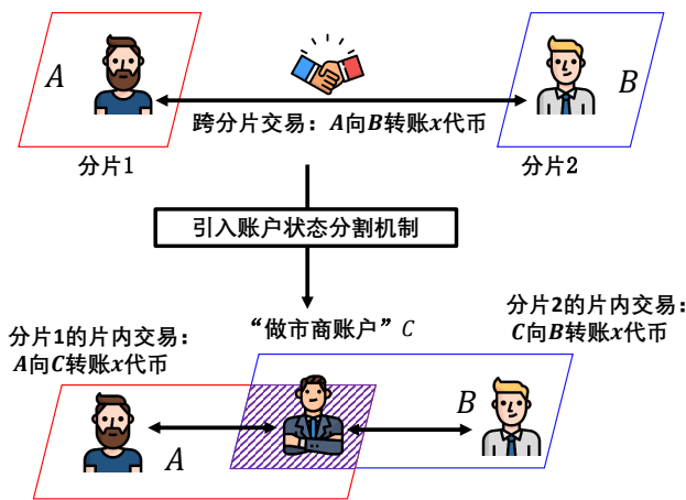
图 2.4: BrokerChain 跨分片协议中的“做市商”交易机制。
