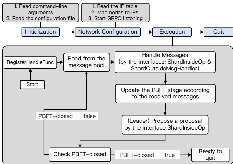
图 7.3: Consensus 节点在 BE-X 中的工作流程。
