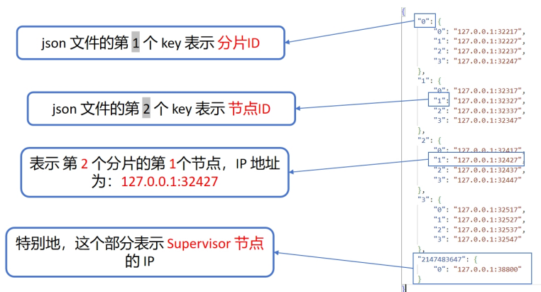
图 4.4: 在 ./ipTable.json 文件中可配置的系统参数。
