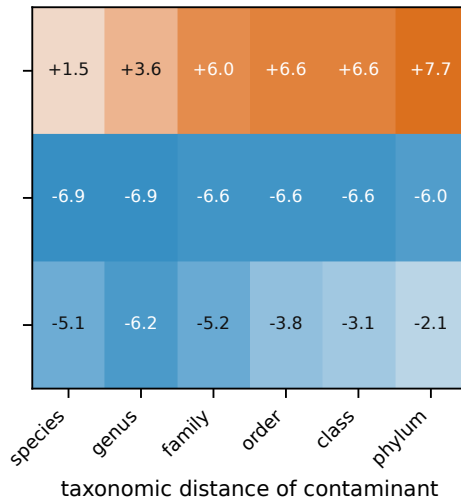
CoCoPyE 0.5.0
