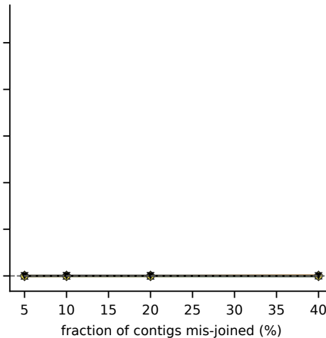
Chimeric mis-joins
