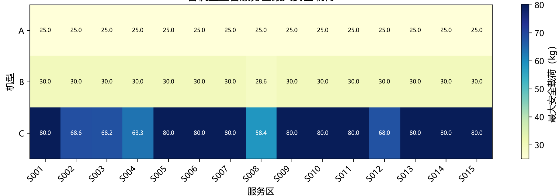
各机型至各服务区最大安全载荷
