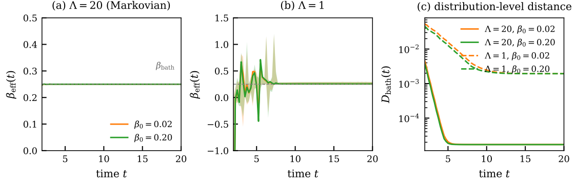
図2 共鳴準位模型による検証 ( \varepsilon_d = 1 , \Gamma_0 = 1 , \beta_{\text{bath}} = 0.25 ). (a) \Lambda = 20 (Markov 的). \beta_{\text{eff}} は \beta_{\text{bath}} に収束し、構造の振幅は 10^{-4} の範囲にとどまる. (b) \Lambda = 1 . \beta_{\text{eff}} は振動し負値もとる. 帯は FDT フィット窓を 2.0–4.0 で変えたときの広がりであり、すべての時刻で二つの初期温度の軌跡の差を上回る. (c) 距離指標 D_{\text{bath}}(t) は両方の場合に単調減少する.
