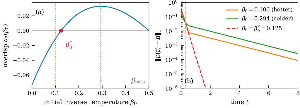
図 1 三状態 Markov 模型による検証 ( E = (0, 1, 5) , \Gamma = (0.3, 2.0, 0.001) , \beta_{\text{bath}} = 0.5 ). (a) a_2 の初期逆温度依存性. \beta_{\text{bath}} のほかに \beta_0^* = 0.125 (赤点) でも零となる. 点線は (b) の初期温度. (b) 定常状態への L^1 距離. 高温側 (橙) は初期に低温側 (緑) より遠いが t = 0.31 (灰破線) で追い越す. 赤破線は \beta_0 = \beta_0^* の強ムペンバ効果.
