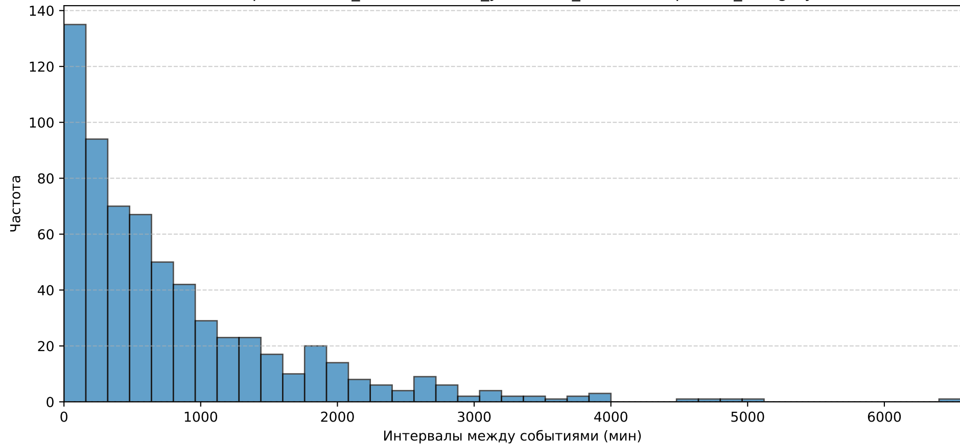
Гистограмма TIME_DIFF — filtered_year-2024_road-Октябрьская_category-2
