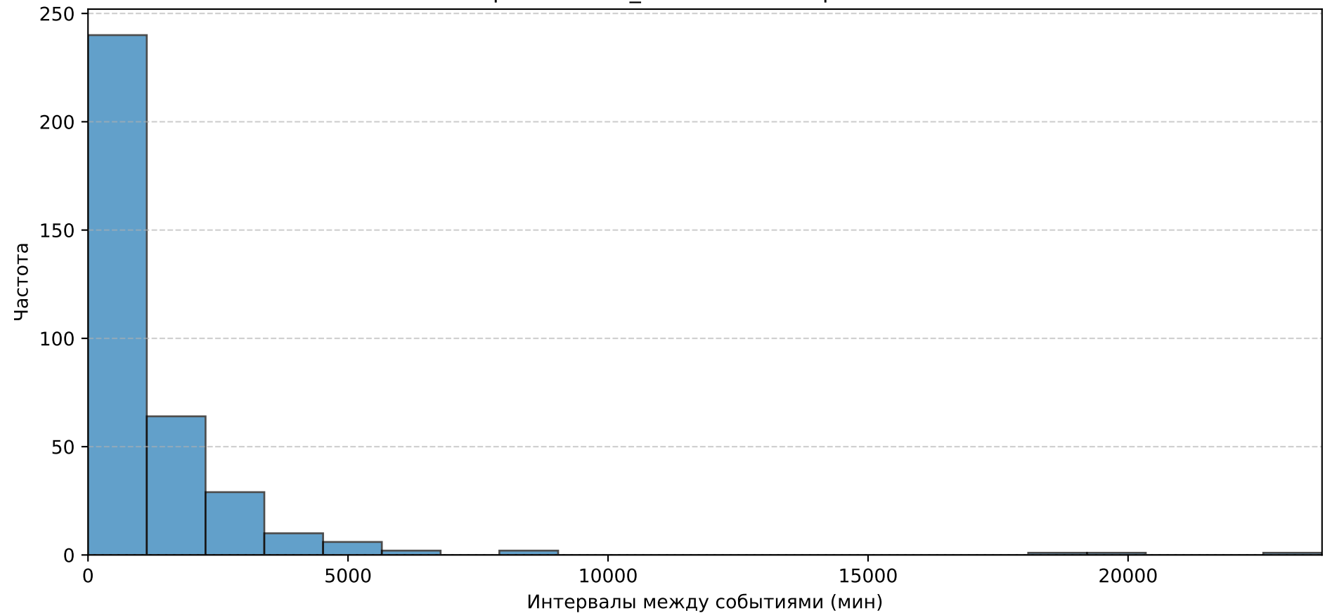
Гистограмма TIME_DIFF — Южно-Уральская-2025
