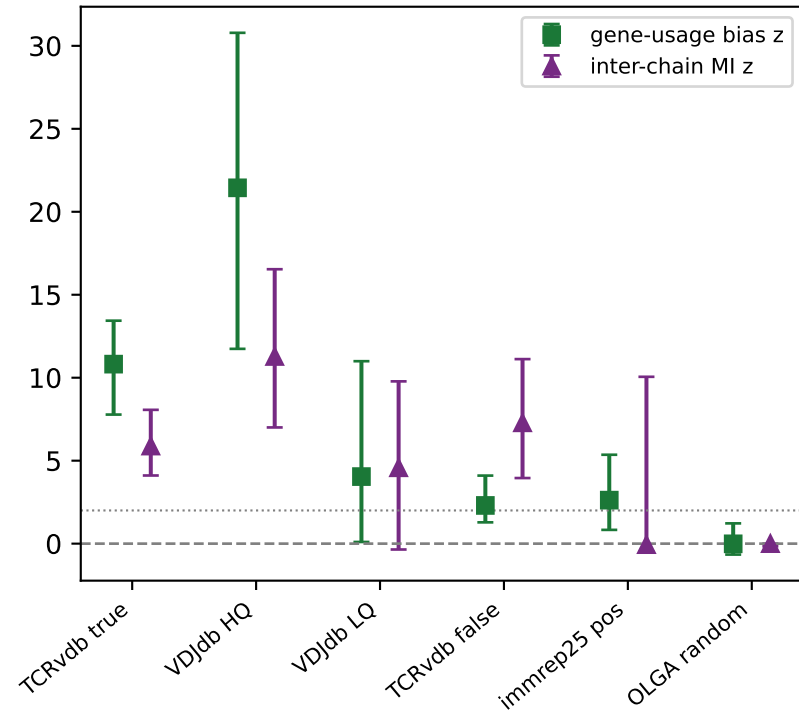
Pairing non-randomness (z vs null)
