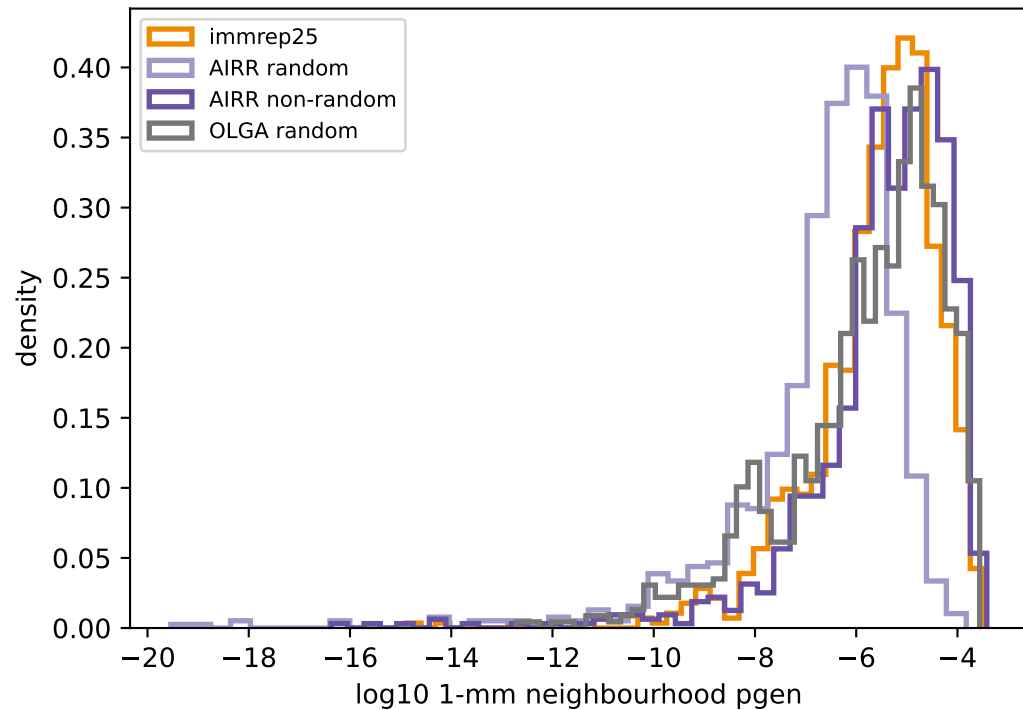
TCR \alpha
