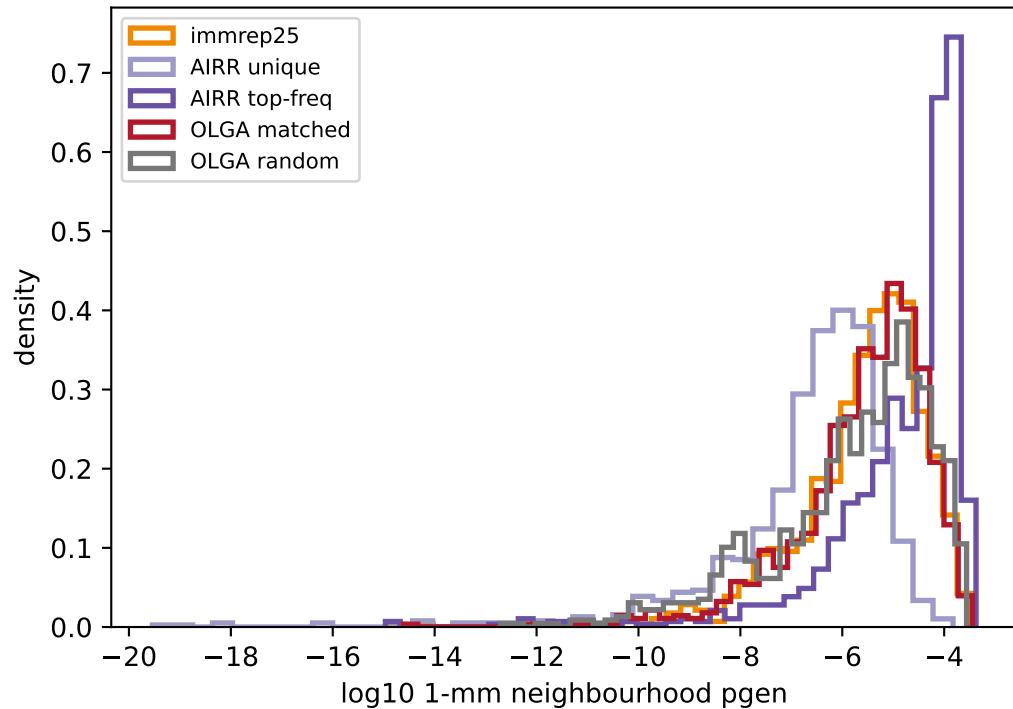
TCR \alpha
