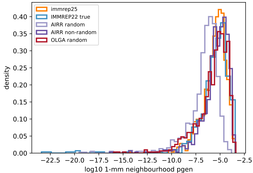
TCR \alpha
