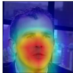
Q30 acc. 0.506
