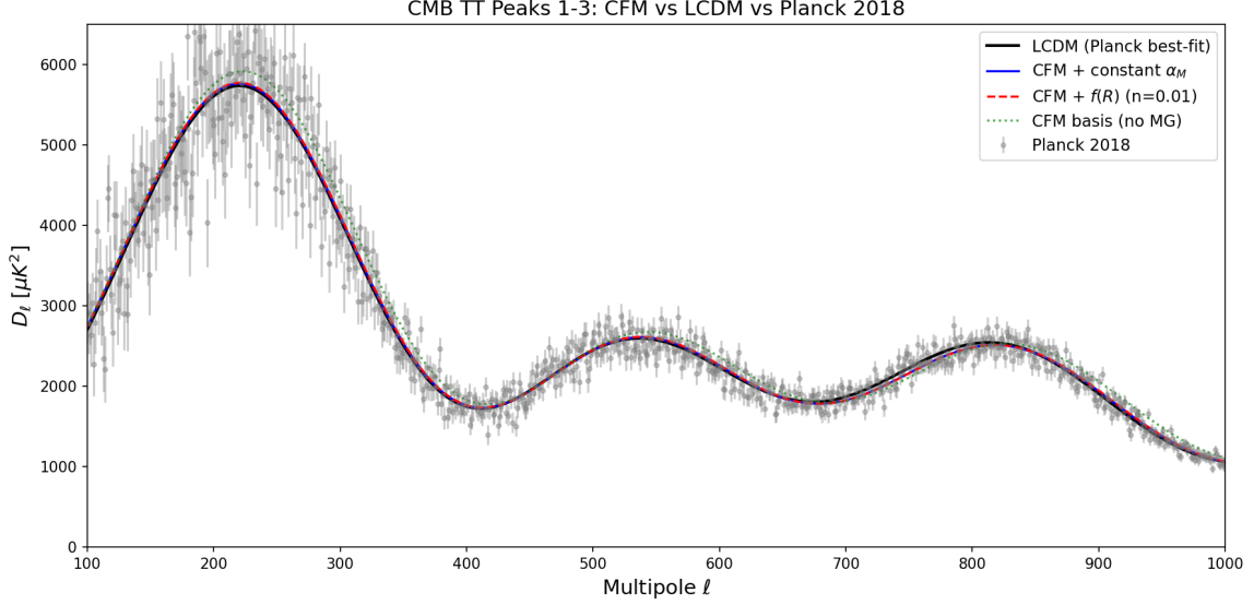
Abbildung 2: Detailansicht der ersten drei akustischen Peaks. Die cfm_fR -Modifikation verschiebt die Position des ersten Peaks durch den frühen ISW-Effekt (gesteuert durch \alpha_M ), ohne die akustische Winkelskala \theta_s zu ändern. Das Verhältnis dritter-zu-erster Peak bleibt erhalten.
