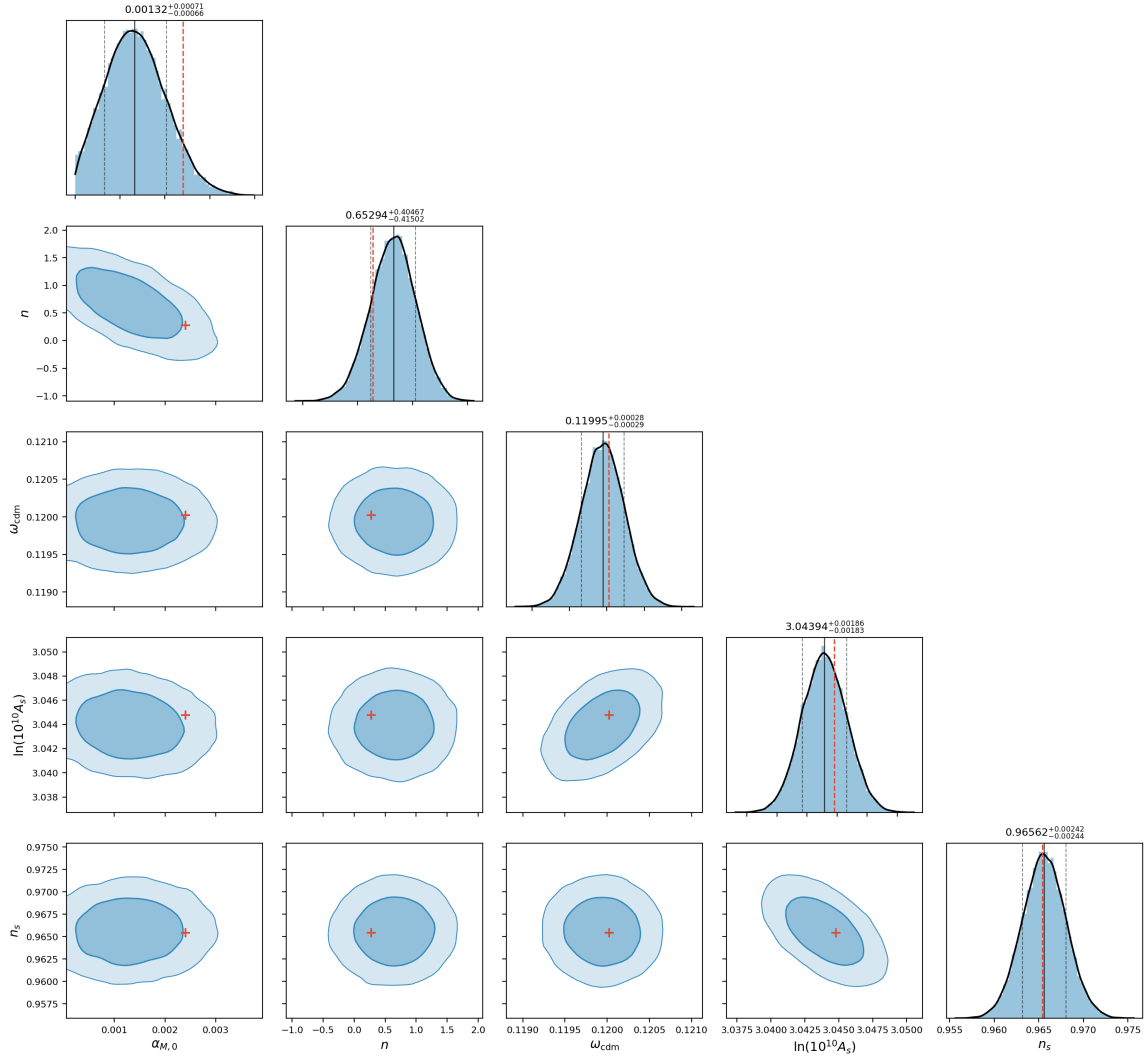
Abbildung 3: Corner-Plot der cfm_fr-MCMC-Posterior (240.000 Samples von 48 Walkern, 5.000 Produktionsschritte). Diagonale Panels zeigen die marginalisierten 1D-Posteriores mit 68%-Kreditätsintervallen (gestrichelte Linien). Off-diagonale Panels zeigen 2D-Konturen bei 68% und 95% Kreditätsniveau mit gefüllten Bereichen. Rote Kreuze markieren den Best-Fit-Punkt ( \chi^2 = 6625,1 , \Delta\chi^2 = -3,7 vs. \Lambda\text{CDM} ). Die Anti-Korrelation \rho(\alpha_{M,0}, n) = -0,61 ist deutlich sichtbar, während alle Kreuzkorrelationen zwischen MG- und Standardparametern |\rho| < 0,08 erfüllen.
