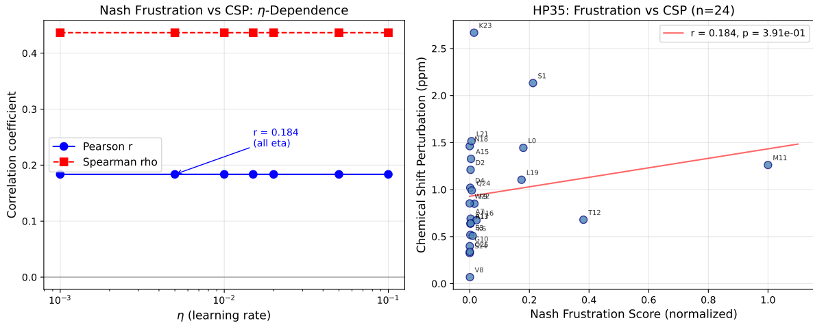
Abbildung 1: Streudiagramm der residuenspezifischen Nash-Frustrationswerte gegen NMR-Chemical-Shift-Perturbation (CSP) für den HP35/1YRF-Benchmark, unter Verwendung von aus BMRB 4428 abgeleiteten HP67-Verschiebungen, die auf die C-terminale HP35-Subdomäne abgebildet wurden. Jeder Punkt repräsentiert einen Rest; die Spearman-Rangkorrelation beträgt \rho_S = 0,44 ( p = 0,033 ). Die Farbkodierung zeigt den Lernraten-Parameter \eta und demonstriert, dass die Frustrations-CSP-Beziehung im geprüften lokalen \eta -Scan invariant ist (alle \eta -Werte fallen auf dieselbe Kurve). Der Ausreißer K23 (hohe CSP, niedrige Frustration) ist auf den Trp-Ringstromeffekt zurückzuführen, nicht auf strukturelle Instabilität.
