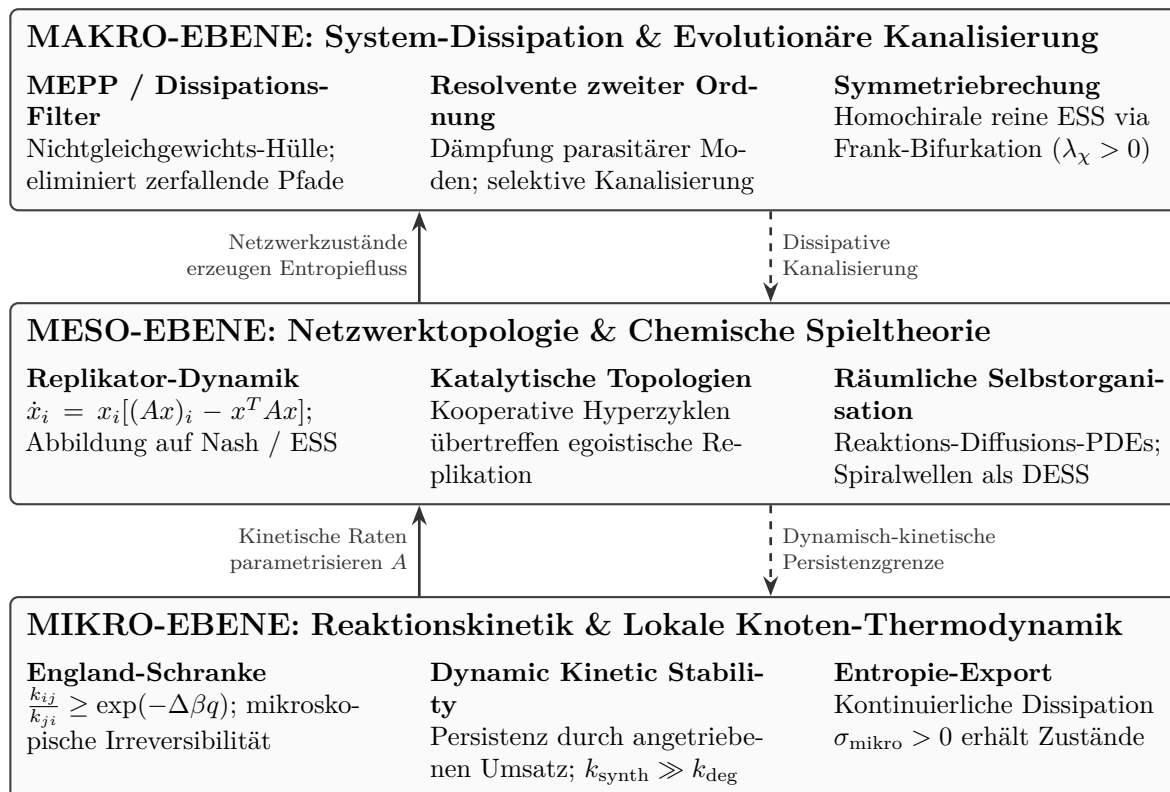
Abbildung 2: Die dreistufige hierarchische Kaskade der Funktionalen Stabilitätstheorie II (FST-II): Verknüpfung der mikroskopischen Reaktions-Thermodynamik (Knoten), der mesoskopischen chemischen Spieltheorie (Netzwerk-Topologie) und der makroskopischen dissipativen Stabilitätsschranke (MEPP/Resolvente).
