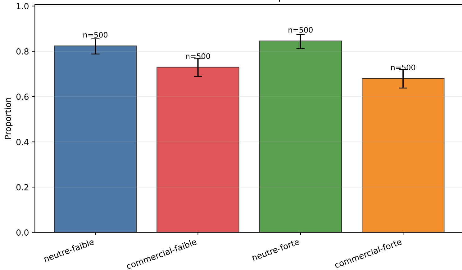
Taux de sélection optimale
