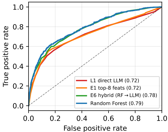
ROC (AUC in legend)
