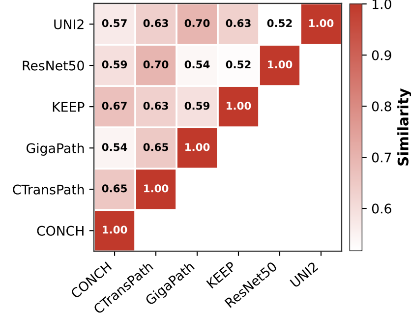
Procrustes
