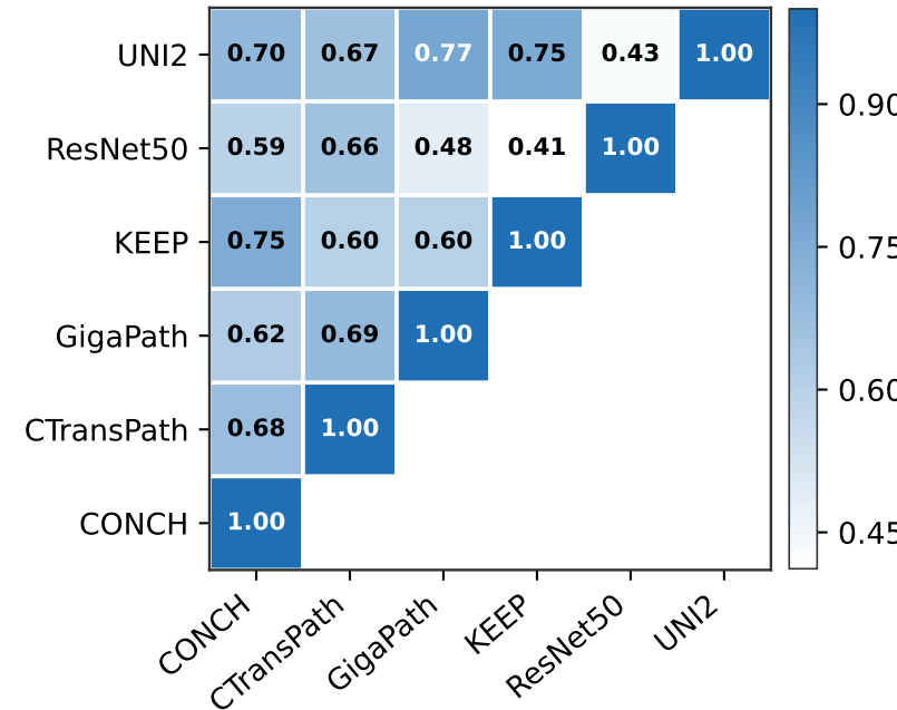
Kernel CKA
