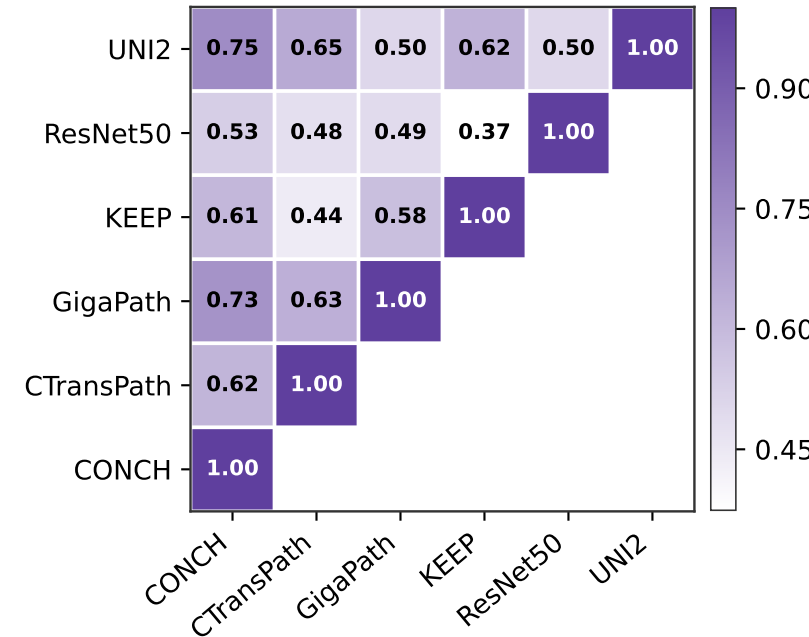
SVCCA
