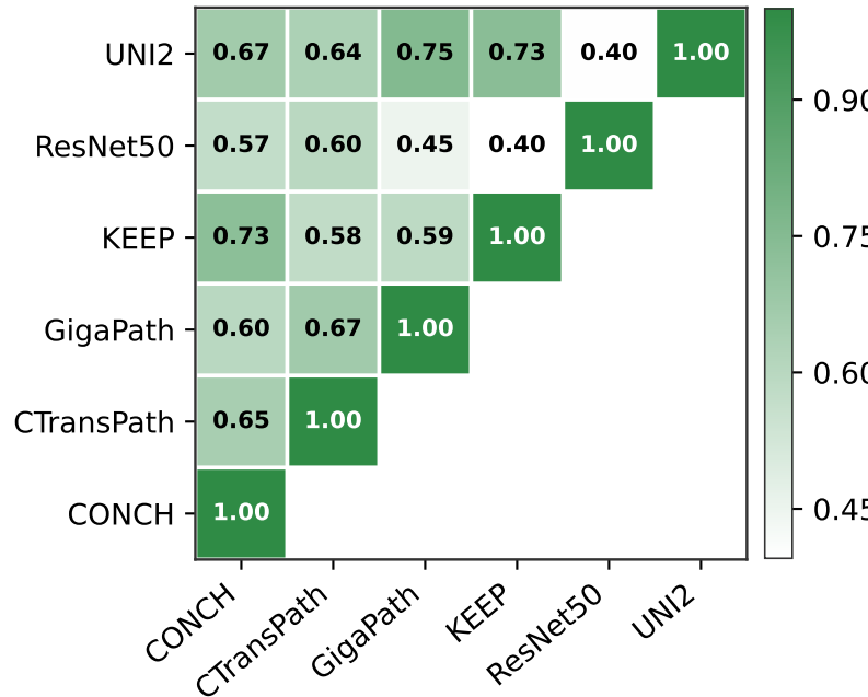
Encoder
