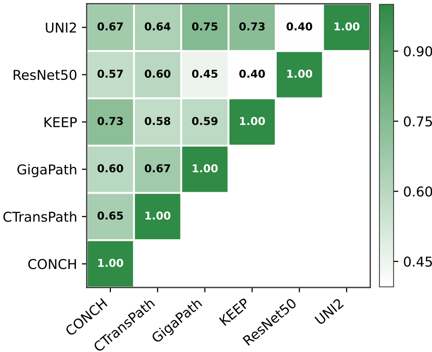
Linear CKA
