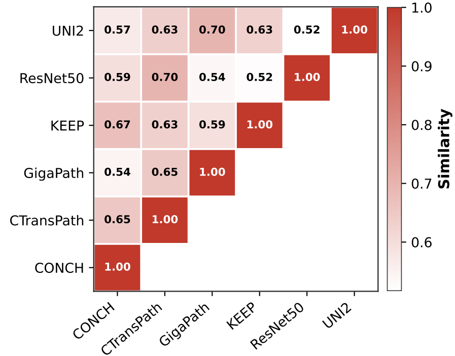
Procrustes
