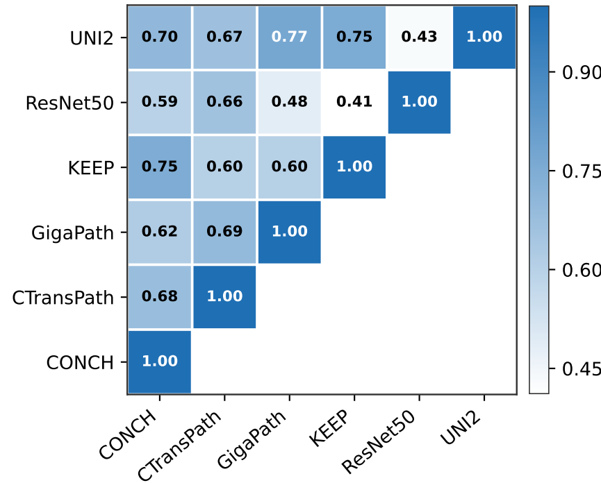
Kernel CKA
