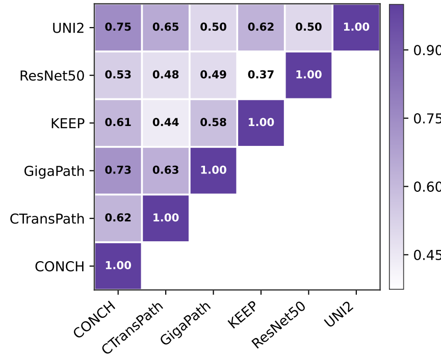
SVCCA
