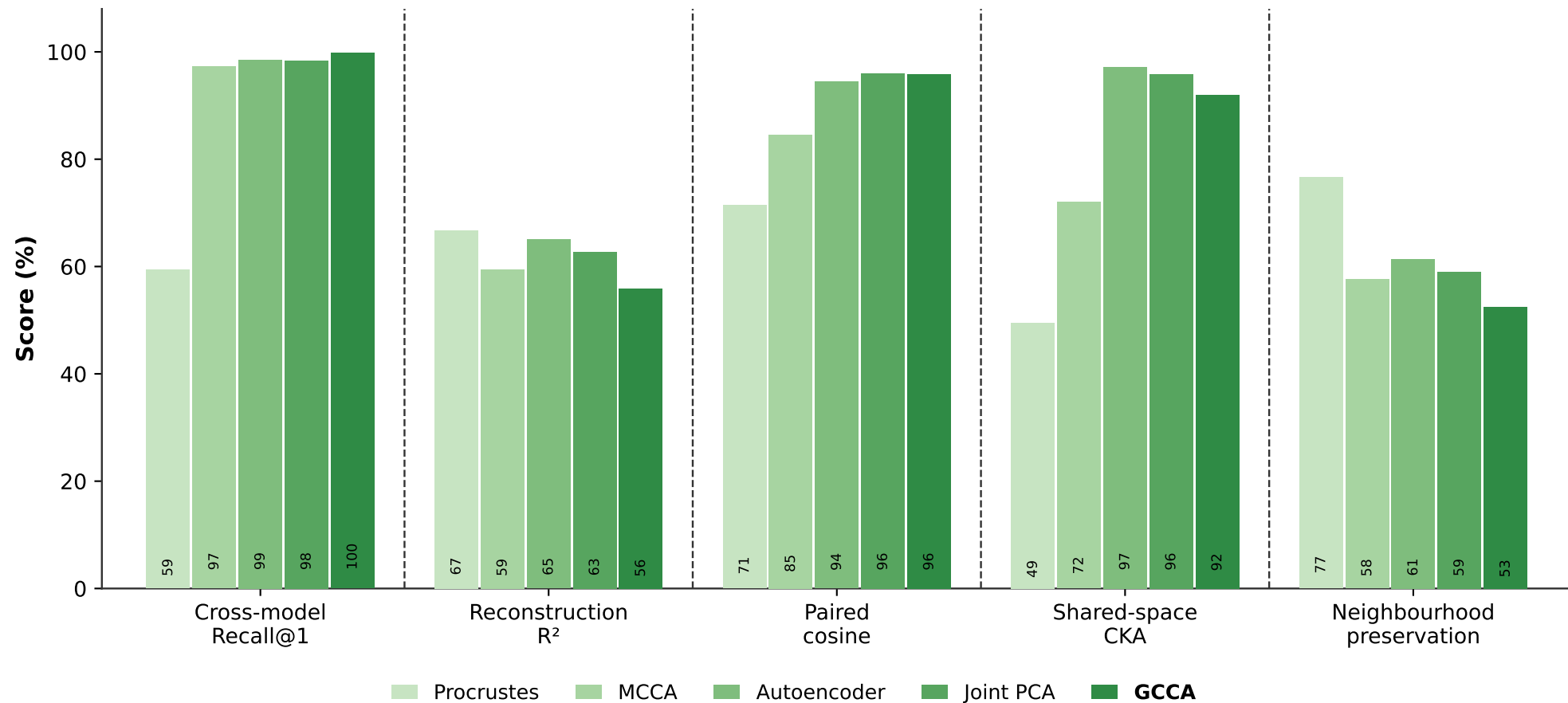
Alignment methods — CPTAC · 20× · 224px (Virchow / GPFM / H-optimus)
