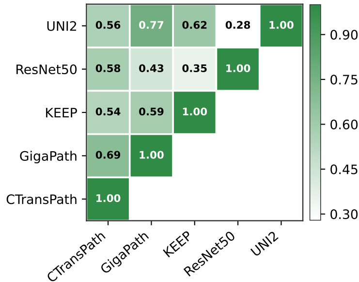
Linear CKA
