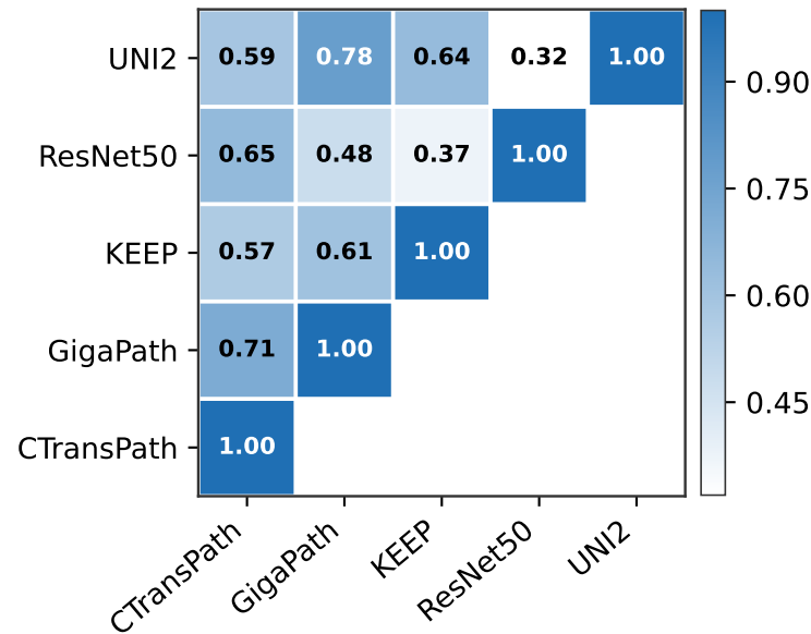
Kernel CKA
