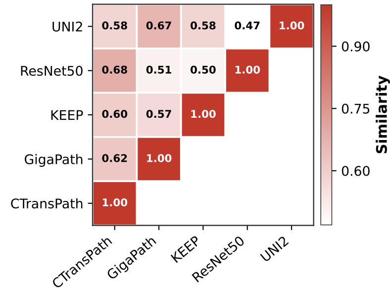
Procrustes
