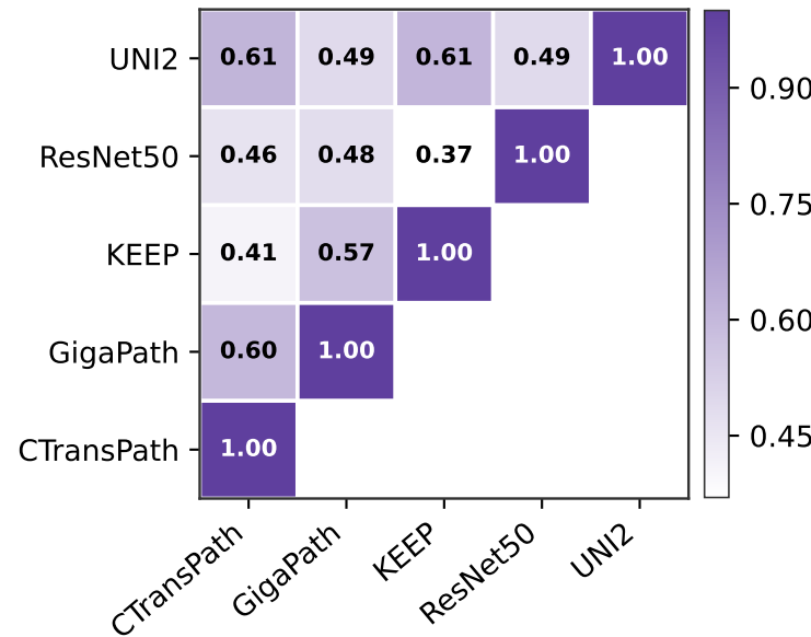
SVCCA
