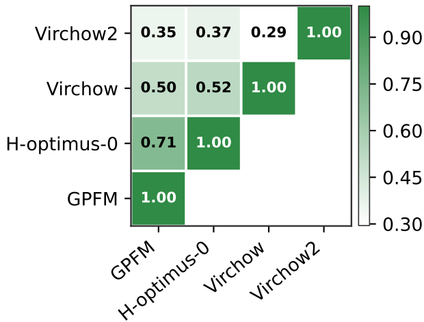
Linear CKA
