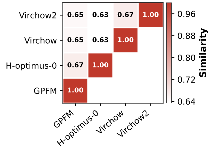
Procrustes
