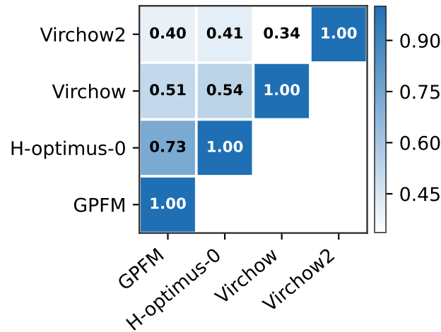
Kernel CKA
