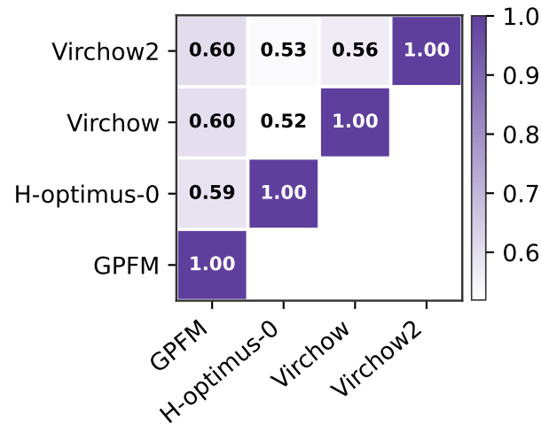
SVCCA
