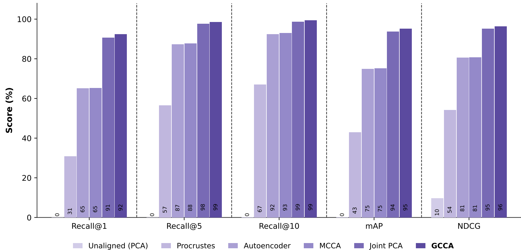
Cross-model retrieval in the shared space · CPTAC · 10× · 256px
