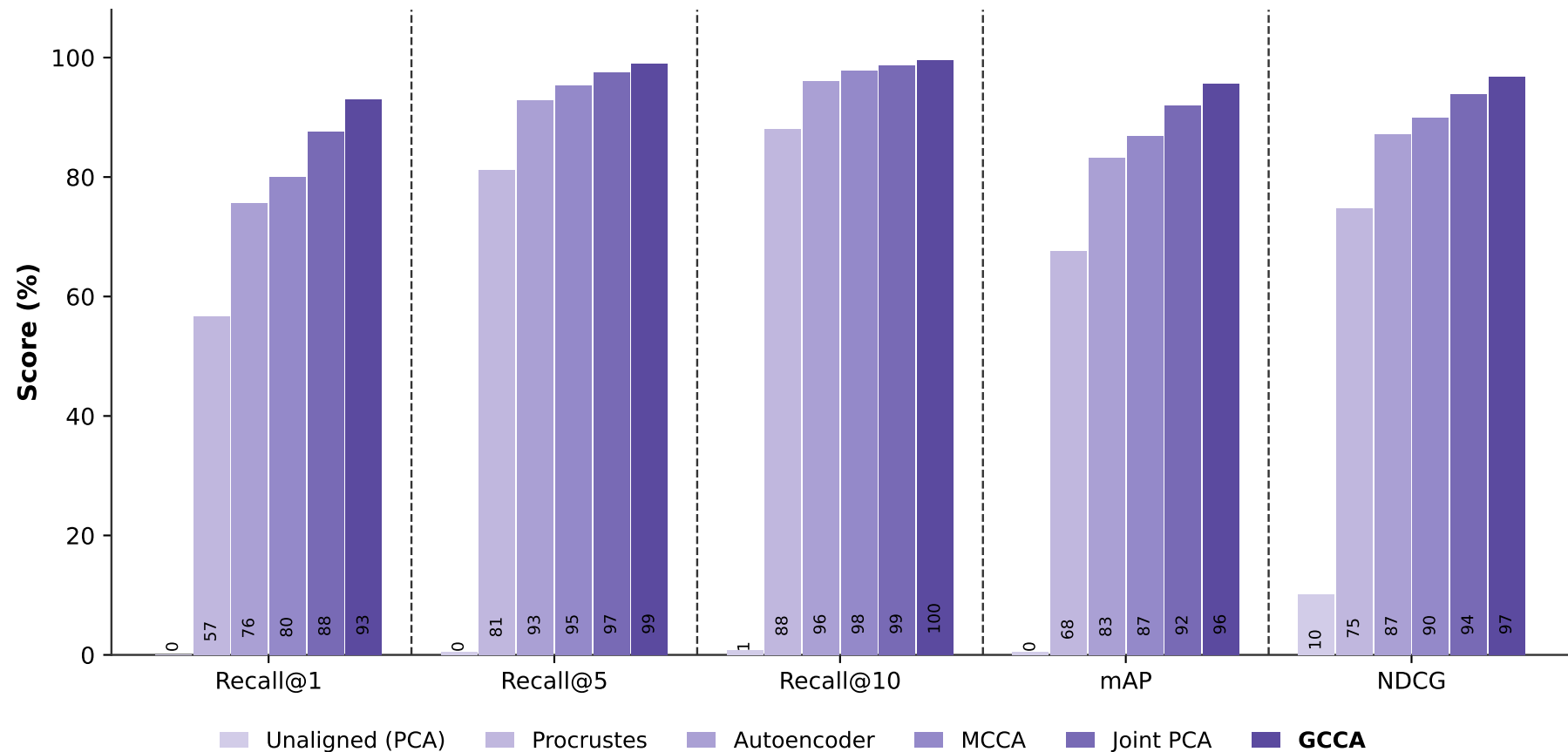
Cross-model retrieval — CPTAC · 10× · 512px (CONCH v1 / v1.5)
