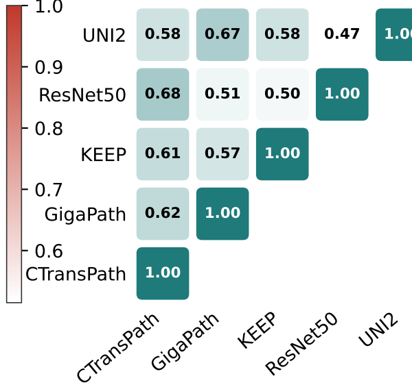
Procrustes
