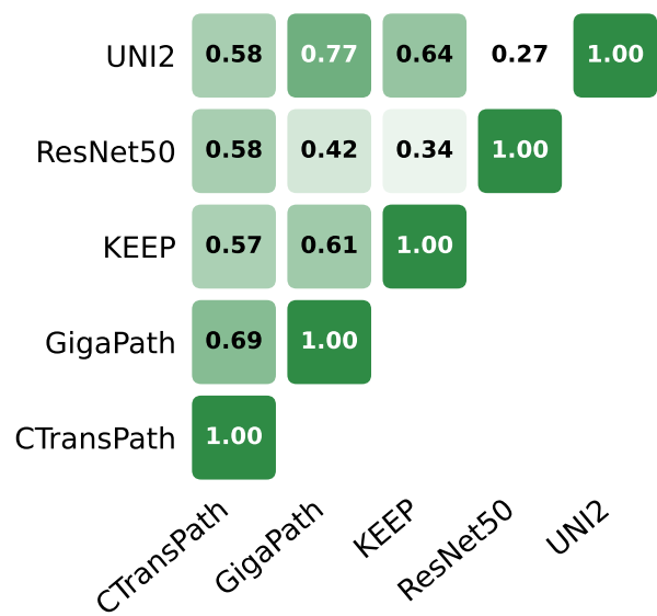
Linear CKA
