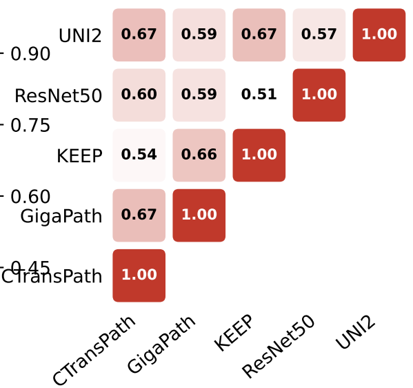
PWCCA
