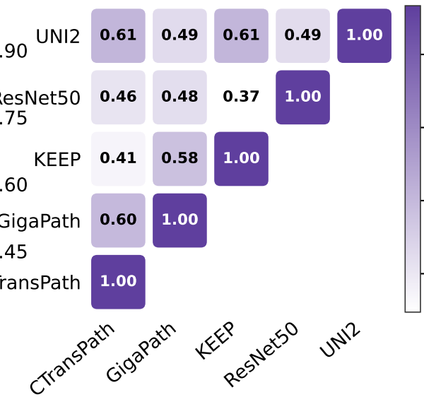
SVCCA
