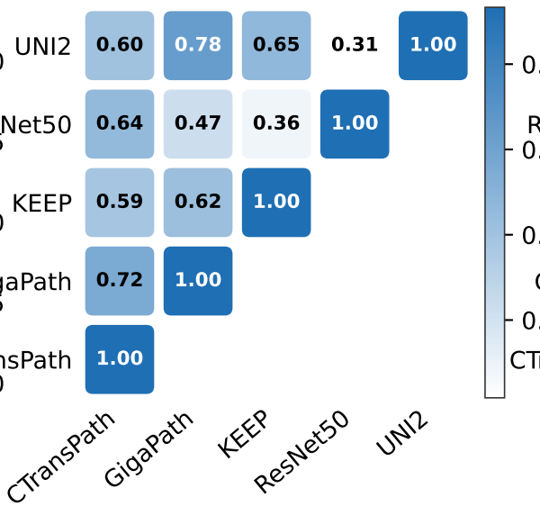
Kernel CKA
