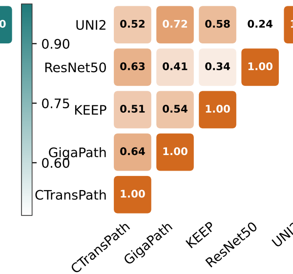
Cosine RSA
