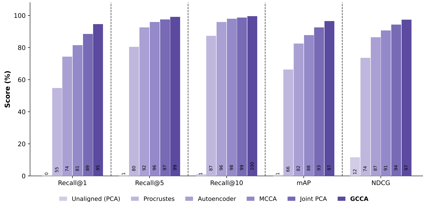
Cross-model retrieval — CPTAC · 20× · 512px (CONCH v1 / v1.5)
